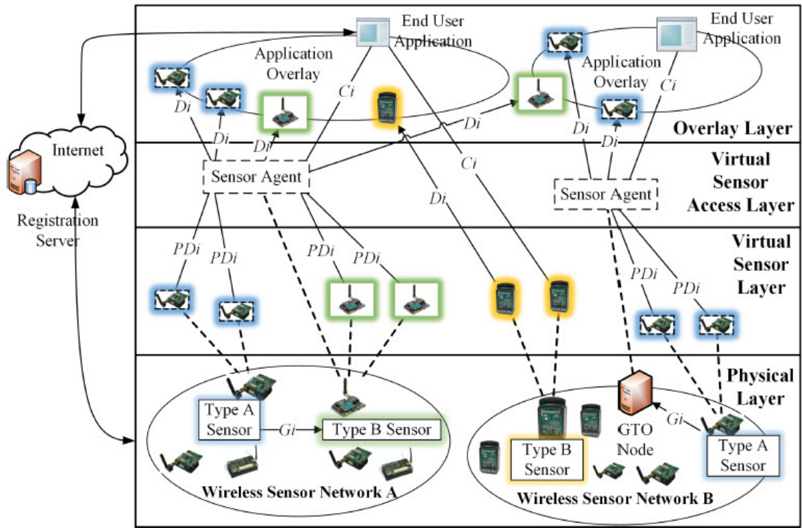
Figure 13: Architecture de réseaux de capteurs virtuels
