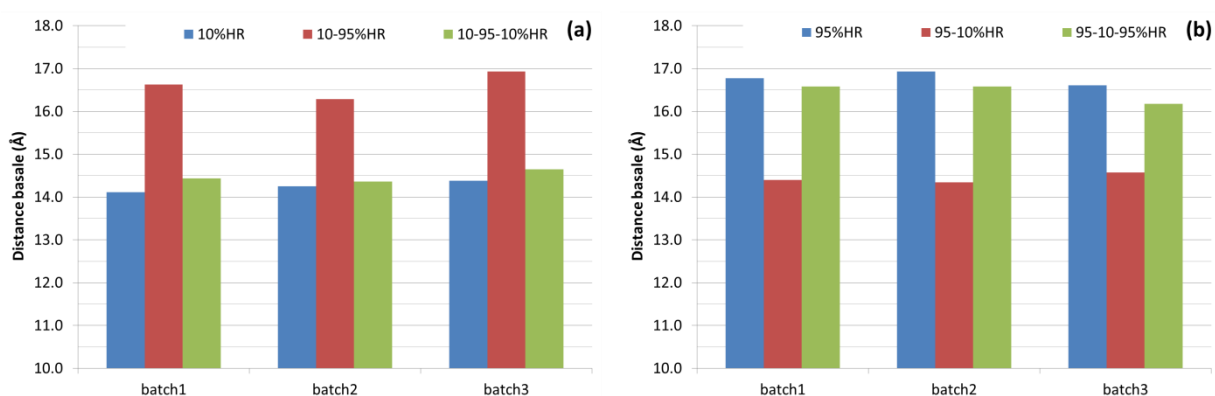
Figure II-5 - Mesure de la distance basale à HR fixée sur 3 batches de montmorillonite non traitée et test de réversibilité de la prise en eau. (a) – 1 er conditionnement à 10% HR puis conditionnement à 95% puis à 10%. (b) – 1 er conditionnement à 95% HR puis conditionnement à 10% puis à 95%.
