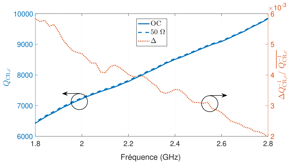
FIGURE 3.10 – Facteur de qualité de la CR dans le cas des différentes charges.
