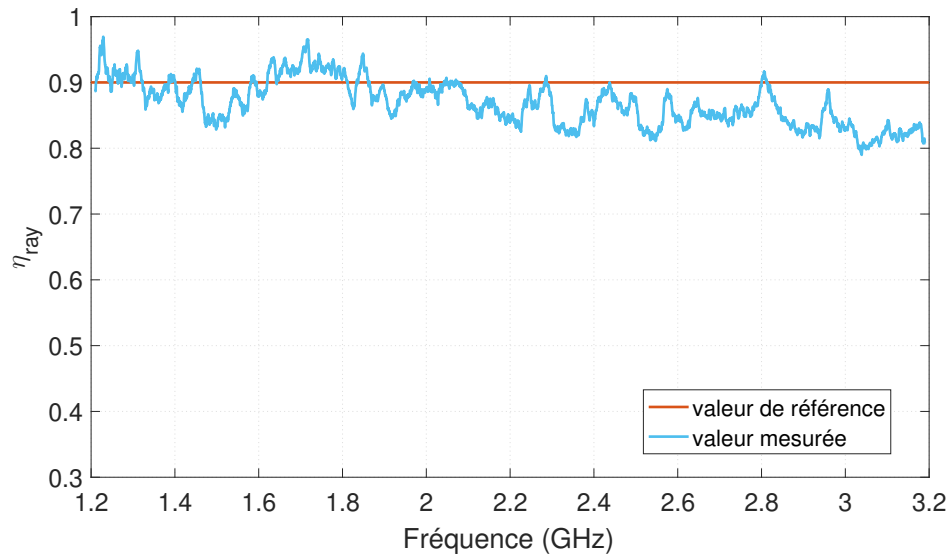
FIGURE 2.8 – Efficacité de rayonnement de l’antenne log-périodique ( \text{Ant}_{\text{ref}} ) comparée à sa valeur supposée fixe et égale à 90%.
