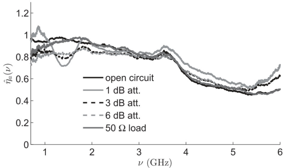
FIGURE 3.3 – Efficacité de rayonnement estimée avec le nouveau modèle proposée dans [122].
