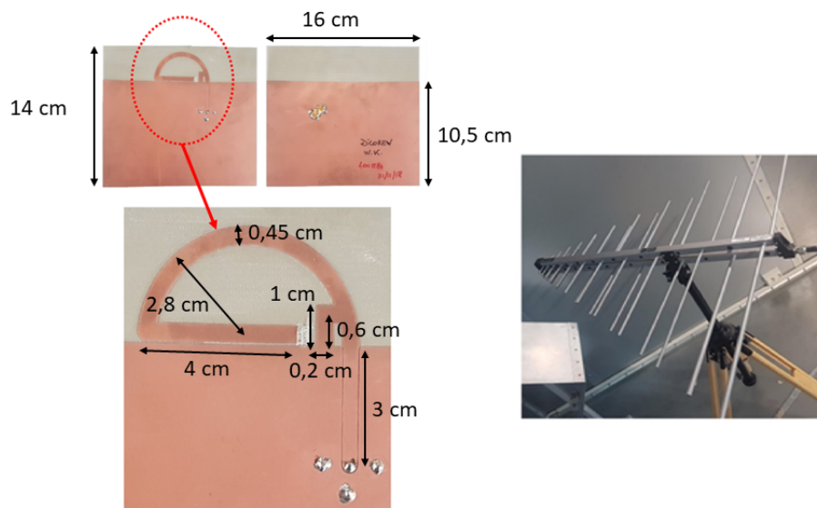
FIGURE 2.23 – Antennes de mesure : antenne patch sous-test (à gauche), antenne log-périodique (à droite).
