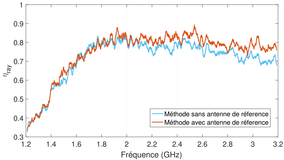
FIGURE 2.7 – Efficacité de rayonnement de l’antenne patch en utilisant les techniques de mesure avec et sans antenne de référence.
