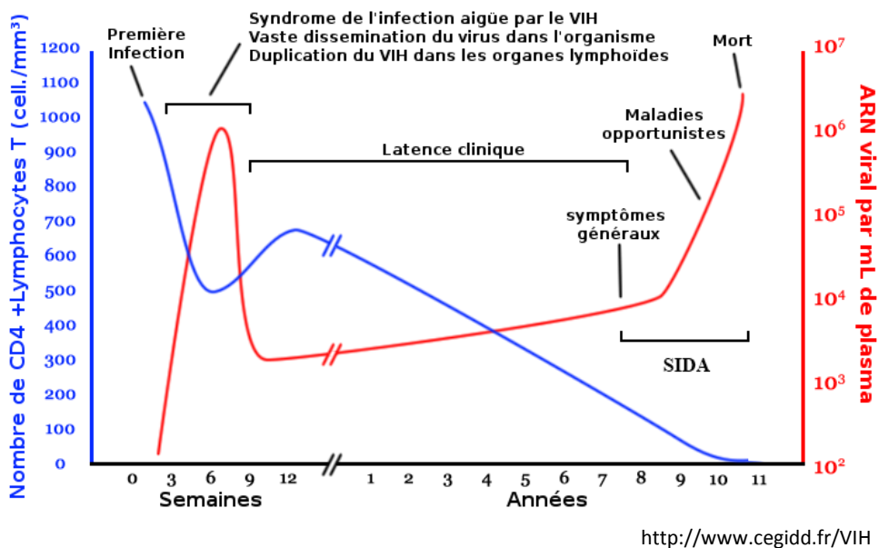
Figure 2 : Evolution clinique de l'infection par le VIH-1. L'infection est caractérisée par 3 phases : primo infection, infection clinique et le SIDA (figure adapté du centre de dépistage et diagnostic). La ligne bleue correspond à l'évolution du taux de lymphocytes T CD_4^+ et la ligne rouge correspond à la charge virale plasmatique.
