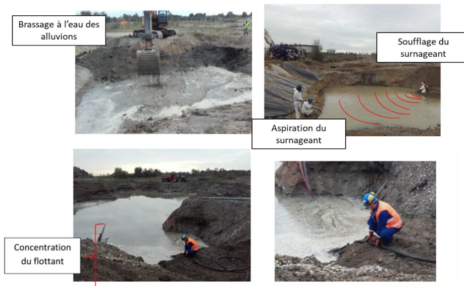
Figure 22 : Synthèse des différentes étapes de dépollution des eaux et des alluvions
