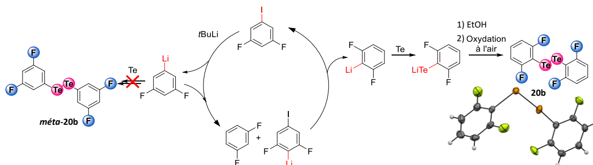
Schéma 82 : Proposition de mécanisme réactionnel pour la formation de 20b avec sa structure cristallographique résolue
