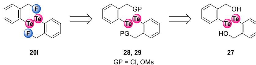
Schéma 85 : Rétrosynthèse de 20I à partir d'un intermédiaire diarylditelluré
