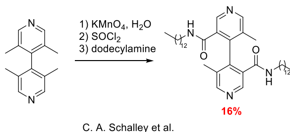
Schéma 23 : Méthode de désymétrisation de 4,4'-bipyridines, du groupe de C. A. Schalley
