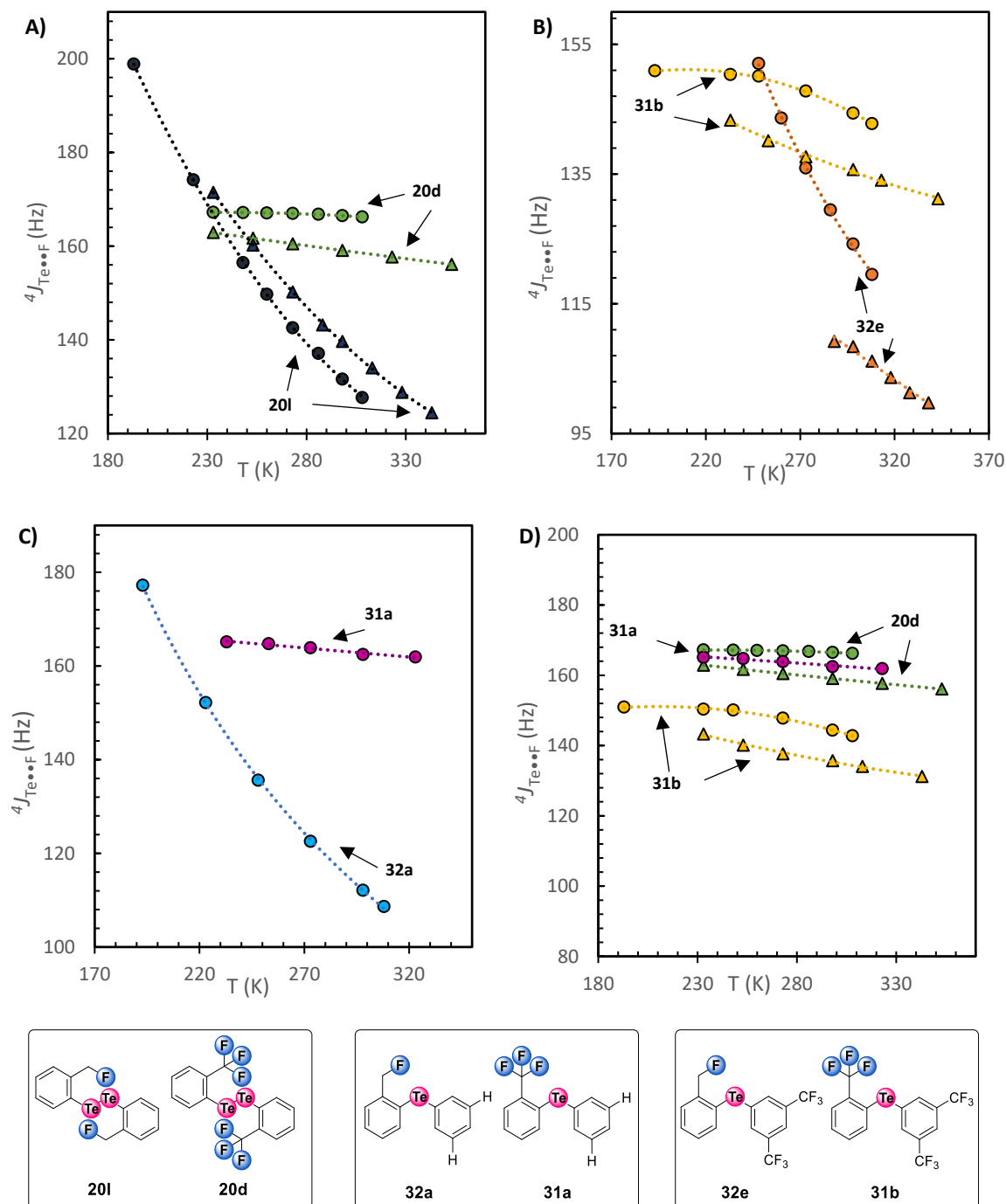
Graphique 9 : Corrélation entre les constantes de couplages observées ^4J_{\text{Te}\cdots\text{F}} et la température (T) ; Légende : \text{CD}_2\text{Cl}_2 (●) et \text{CD}_3\text{CN} (▲) pour 20l (●/▲), 32a (●/▲), 31b (●/▲), 20d (●/▲), 32e (●/▲), 31a (●/▲)
