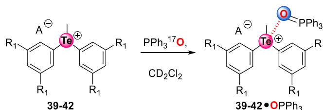
Schéma 118 : Réaction de complexation étudiée en solution, entre les sels de telluronium substitués avec différents motifs R_1 et contenant différents anions A^- , et OPPh_3 dans CD_2Cl_2 à 25 °C.
