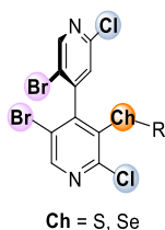
Schéma 148 : Le motif de 4,4'-bipyridine chalcogénée étudiée en organocatalyse
