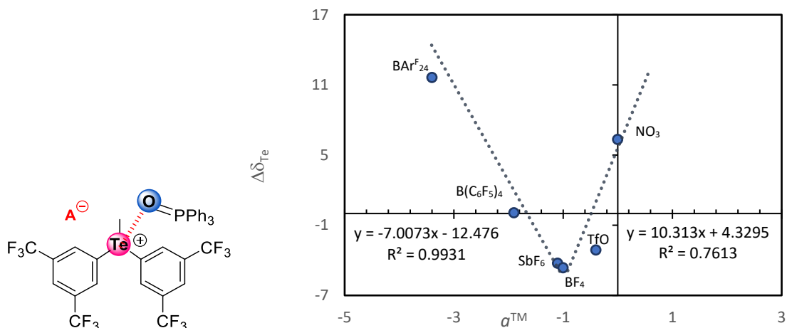
Graphique 19 : Corrélations entre \Delta\delta_{Te} (ppm) et \alpha^{TM} \Delta\delta_o (ppm) dans la série 41a-f, dans CD_2Cl_2 à 25 °C
