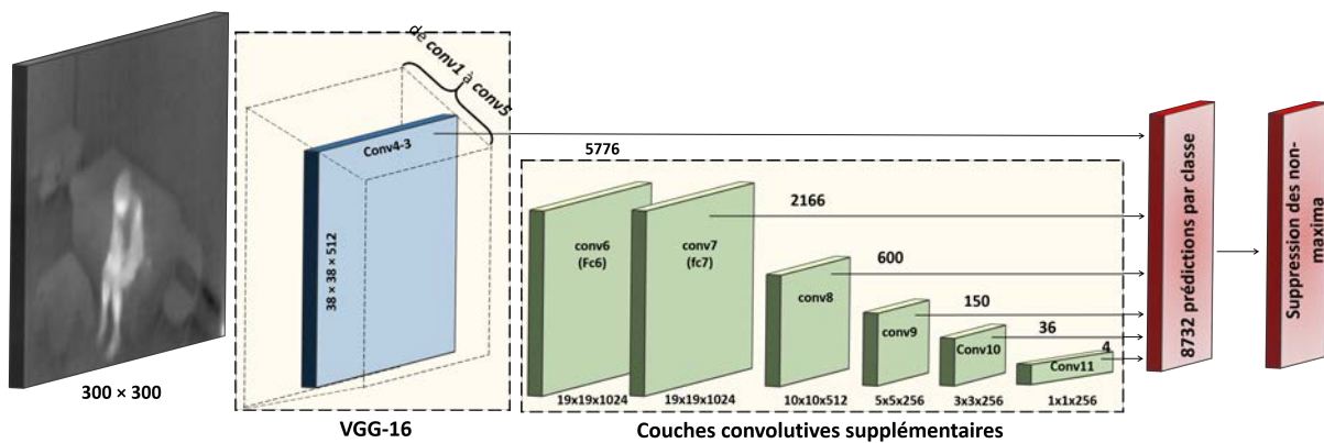
FIGURE 7.5 – L'architecture globale du réseau SSD.
