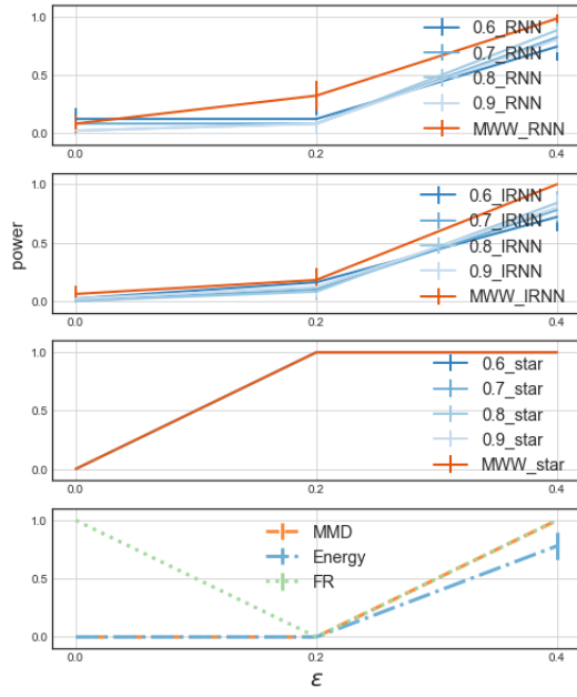
a. (S2), d = 3
