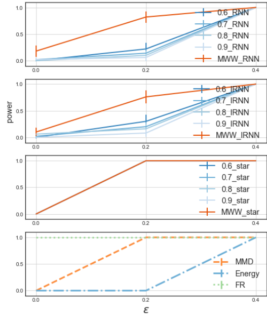
b. (S2), d = 20
