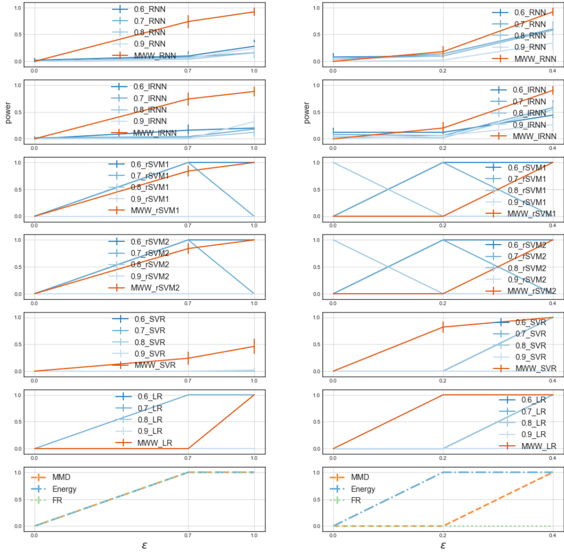
a. (BL), \theta = 3
