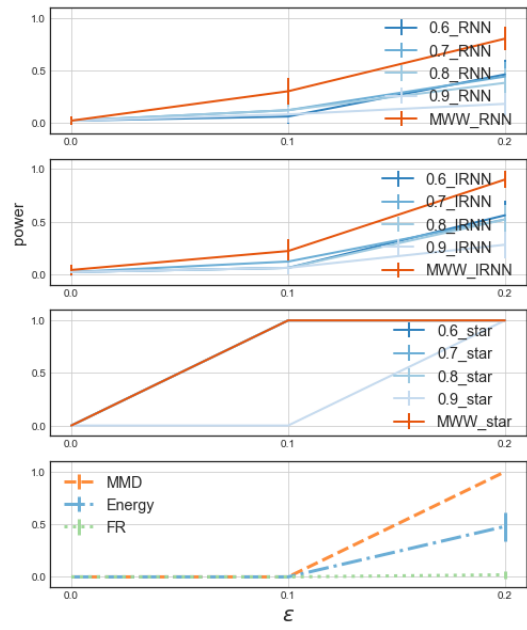
d. (S3), d = 20
