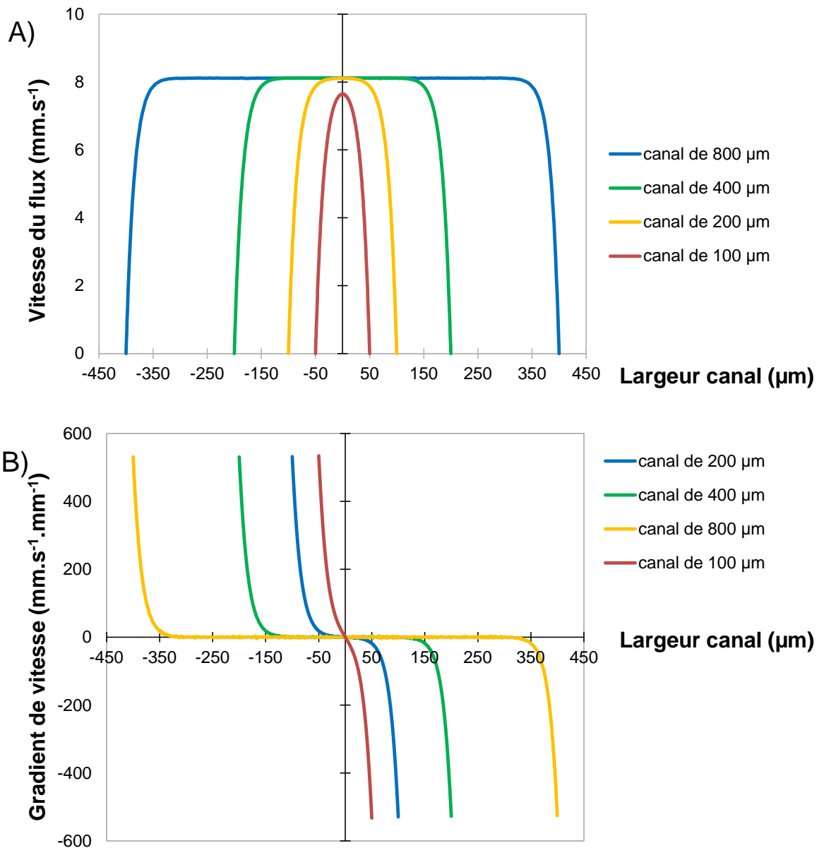
Figure.53 : A) Profil de la vitesse du flux dans des canaux de différentes largeurs avec une pression imposée afin d'avoir une vitesse de 8 \text{mm}\cdot\text{s}^{-1} . B) Gradient des profils de vitesses de A). Tous deux simulés sous COMSOL Multiphysics.
