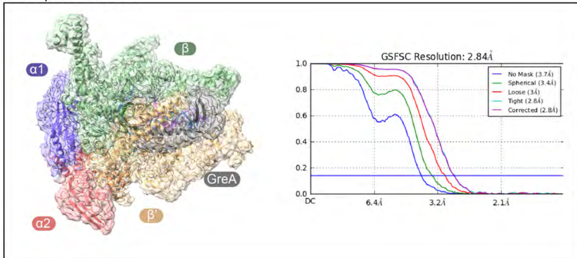
a. Complexe avec GreA
