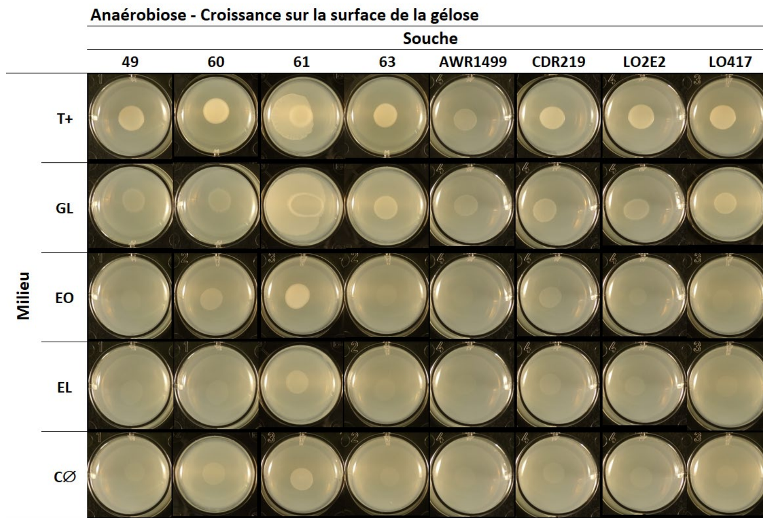
Figure 2.S1 (Suite). Photos des cultures de seize souches de Brettanomyces bruxellensis sur différents milieux gélés variables en source de carbone avant lavage (Croissance sur la surface de la gélose) après 7 jours d'incubation en aérobiose ou anaérobiose. T+ : milieu complet ; GL : glucose limité ; EO : éthanol optimal ; EL : éthanol limité ; CØ : sans glucose ni éthanol.
