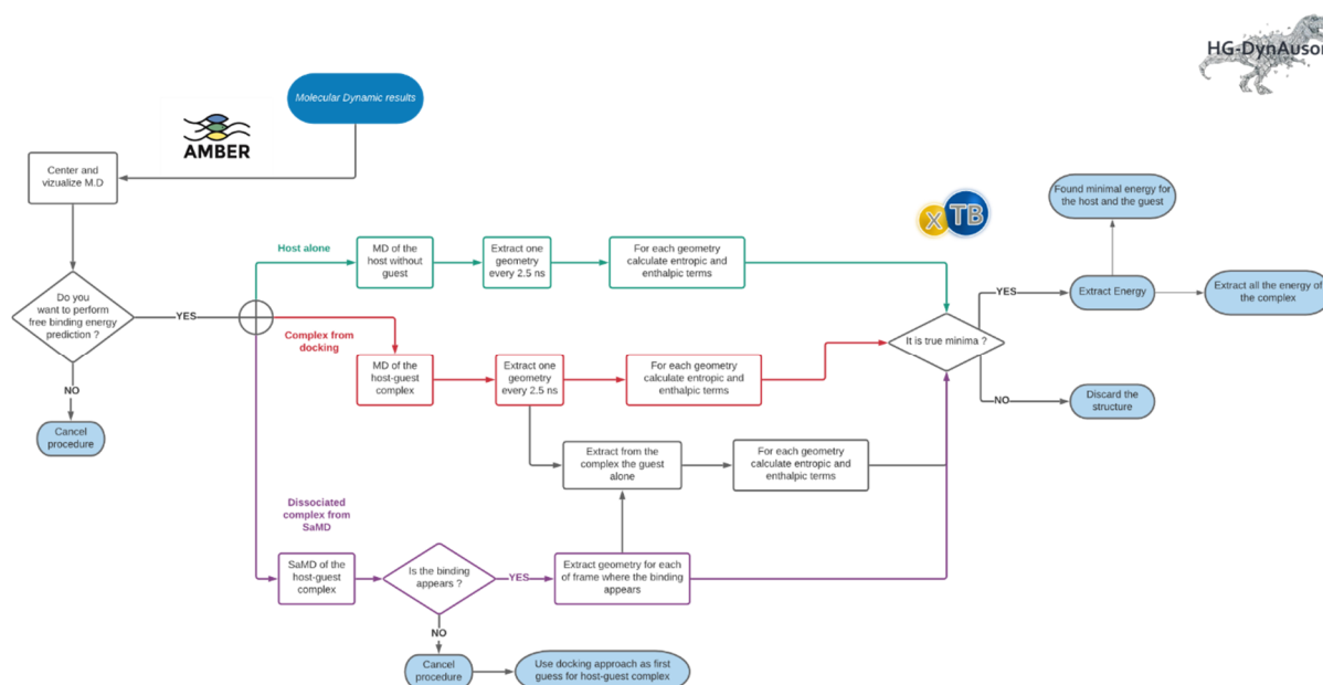
Figure 0. 7 : vue d'ensemble du module 03 de la plateforme HG-DYNausor dédiée au calcul des énergies libres de Gibbs
