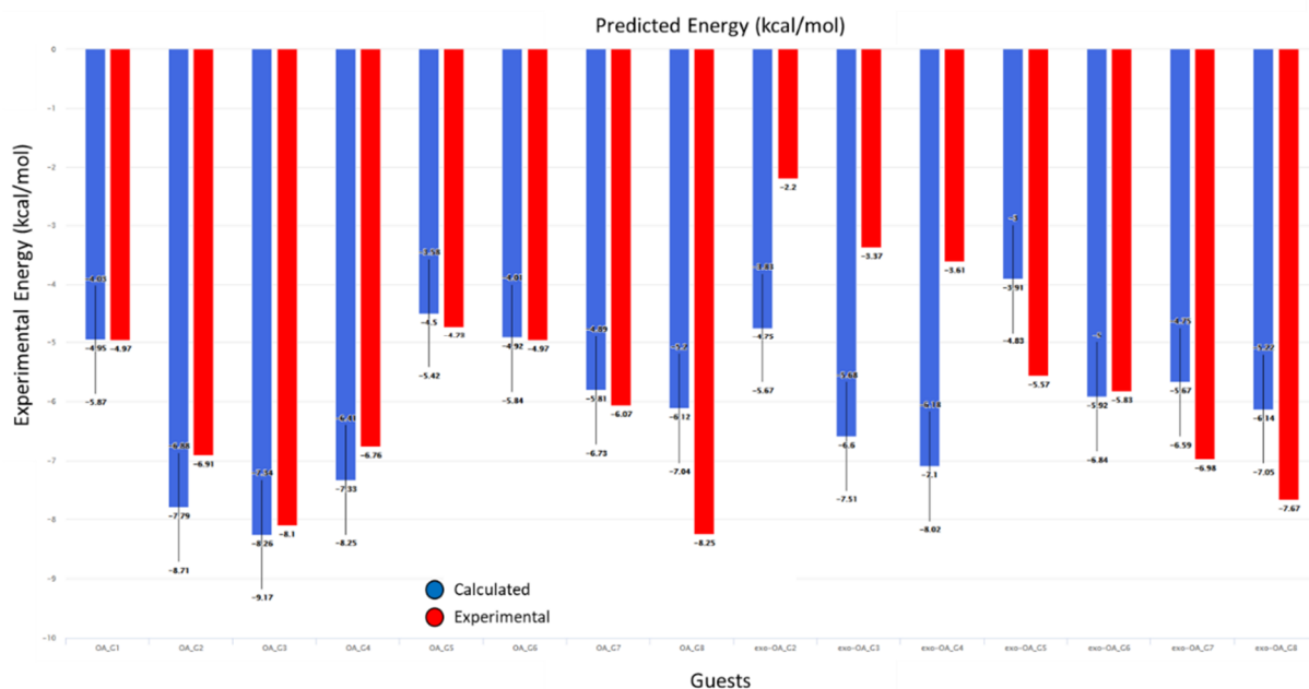
Figure 0. 13 : comparaison des valeurs expérimentales et prédites pour les énergies libres de Gibbs. (A) Graphique de corrélation, la zone en verte, représentant le seuil de +1/-1 kcal/mol. Les symboles indiquent la nature des invités et chaque prédiction possède une couleur différente. (B) Histogramme de la prédiction, avec en bleu les valeurs prédites et en rouge les valeurs expérimentales. Les barres d'erreurs reflètent l'erreur moyenne du modèle (RMSE).
