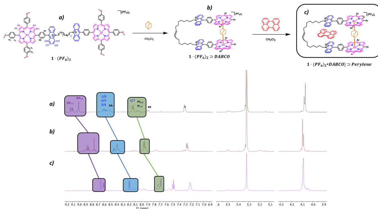
Figure 117: Stacked ^1\text{H} NMR spectra (CDCl 3 , 298 K, 500 MHz) of a) 1 \cdot (PF_6)_2 b) 1 \cdot (PF_6)_2 \cdot DABCO and c) [1 \cdot (PF_6)_2 \cdot DABCO] \supset Perylene
