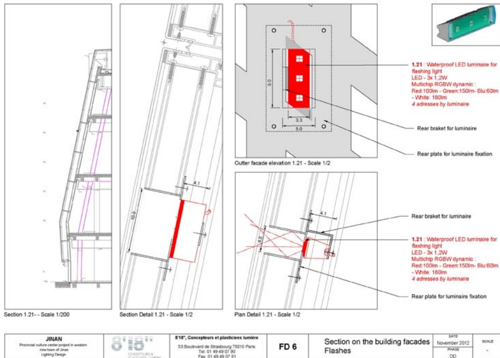
Figure 30. Coupe – détail de l'installation 3
