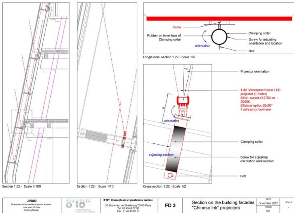
Figure 29. Coupe – détail de l'installation 2
