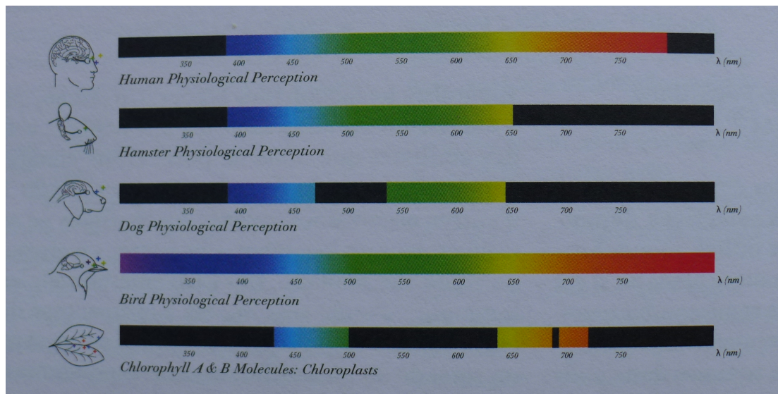
Figure 3 Les spectres visibles de l'humain, des animaux domestiques, oiseaux et plantes vertes 52
