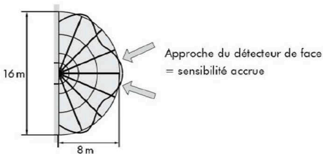
Figure 17. Schémas d'explication sur la zone de sensibilité pour le système de détection de présence
