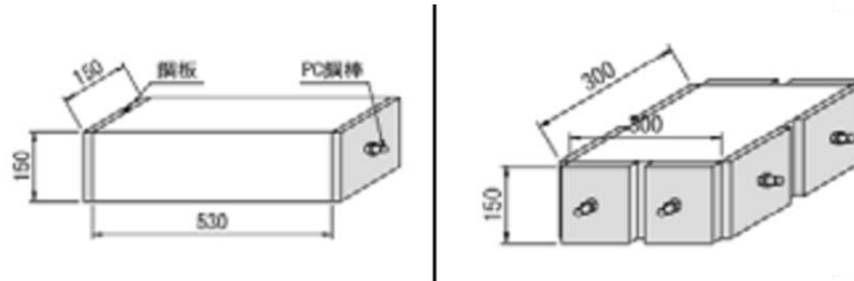
Figure II-8 Schéma des appareillages pour le cas armé uniaxialement et bi axialement [Tasukada et al., 2010]
