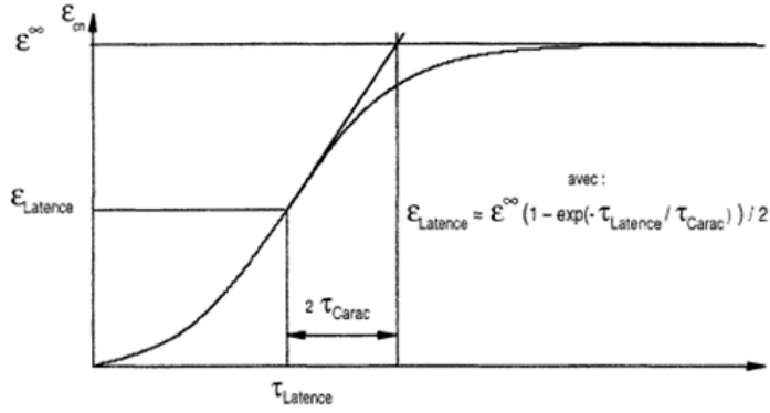
Figure II-53 Equation de la courbe d'expansion proposée par [Larive 1998]
