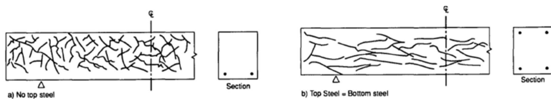
Figure II-41 Orientation de la fissuration par la présence d'armature [ISE, 1992]
