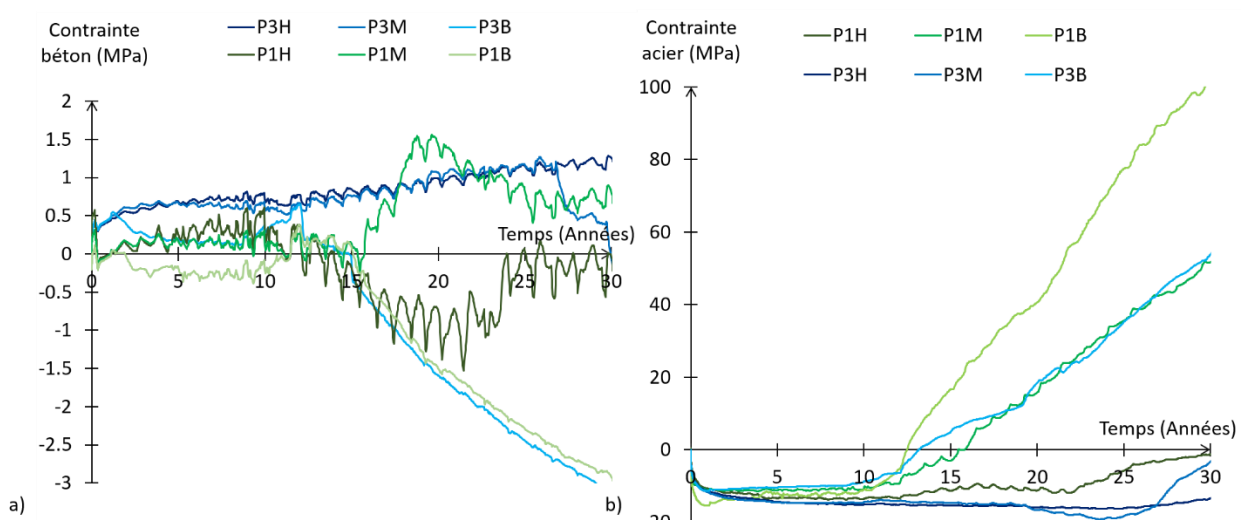
Figure II-22 Evolution des contraintes radiales du radier, a) Dans le béton, b) Dans les armatures
