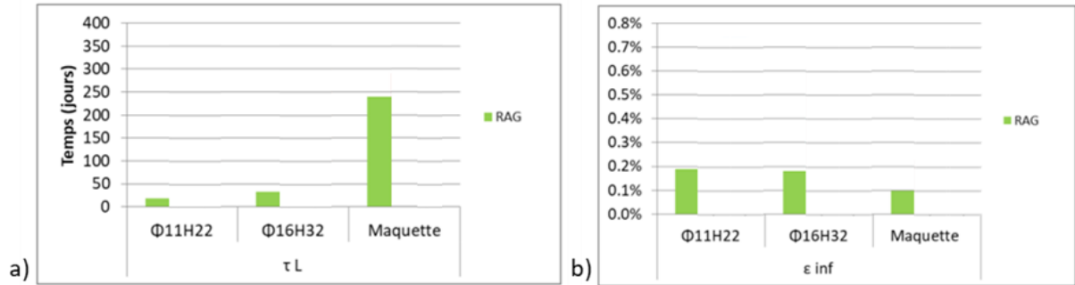
Figure II-49 Comparaison pour les trois corps d'épreuve a) Des temps de latence, b) Des déformations finales [Jabbour, 2019]
