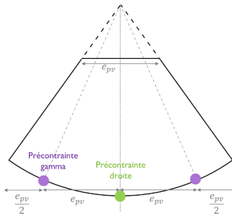
Figure I-3 Schéma représentatif pour la définition du maillage dans le plan X-Y
