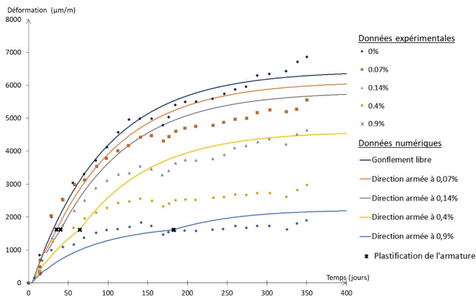
Figure II-7 Evolution des déformations dans la direction armée pour différents ratios d'armature [Koyanagi et al., 1998]
