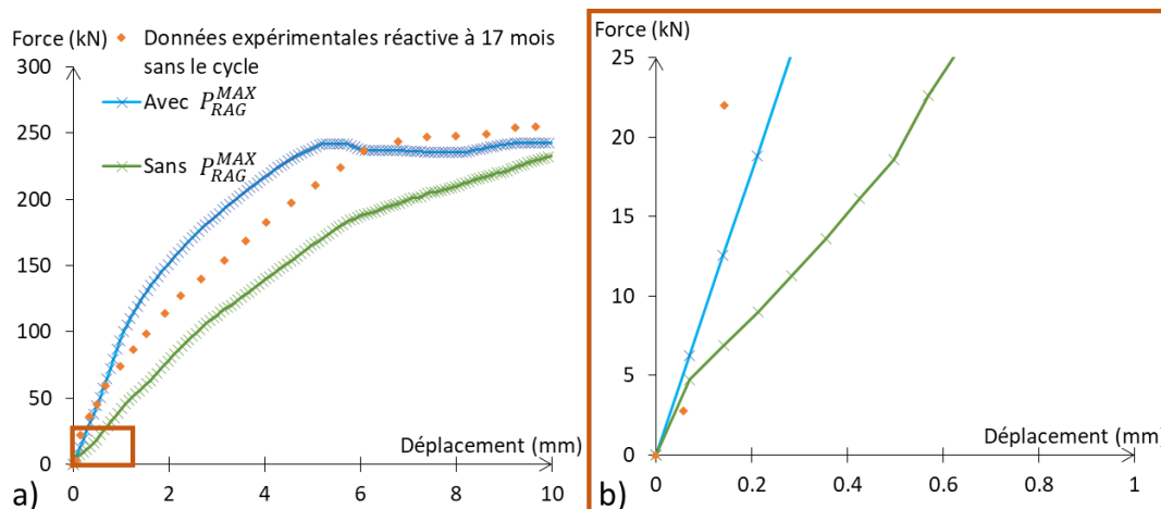
Figure II-6 Comparaison des réponses structurales avec et sans l'usage de la pression maximale, a) Evolution globale, b) Focus sur l'évolution initiale
