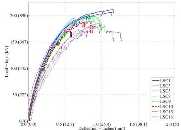
Figure II-46 Résultats des essais de flexion trois points [Bracci et al., 2012]
