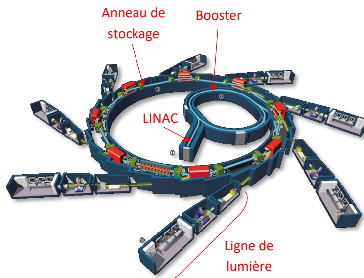
Figure II.30. Représentation d'un synchrotron [159].
