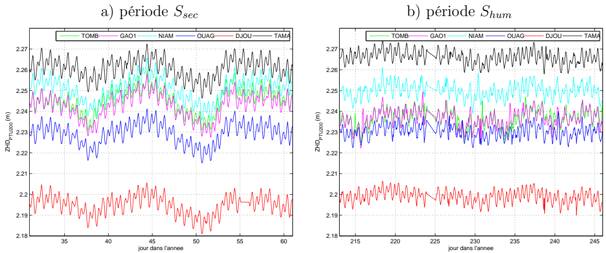
FIGURE 4.8 – ZHD a priori obtenus à partir des mesures PTU200 sur les périodes S_{sec} (a) et S_{hum} (b) pour les stations AMMA.
