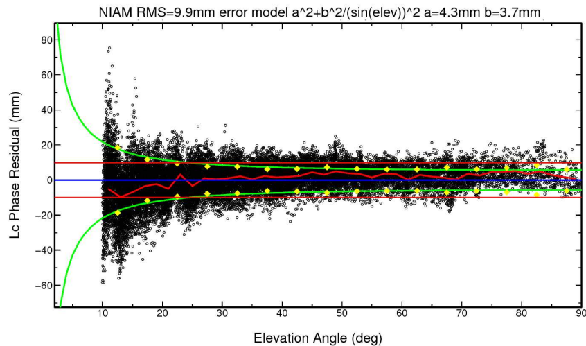
FIGURE 2.2 – Résidus sur les mesures de phase (en noir) en fonction de l'élévation obtenus pour la station de Niamey (Niger) lors du traitement du jour 213 de l'année 2006. Les paramètres du modèle d'erreur de la mesure GPS \sigma_{mes}(elev) = \sqrt{a^2 + b^2/\sin^2(elev)} sont estimés à 4,3 mm pour a et 3,7 mm pour b . En vert, l'enveloppe associée au modèle d'erreur, en rouge la moyenne mobile des résidus de phase, en bleu l'axe \epsilon_{p,\Phi}^e = 0 .
