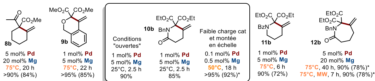
Figure 5: Produits de cyclisations >5-exo obtenus avec le système multi-coopératif
