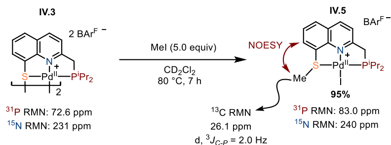
Scheme 16: Illustration du caractère bifonctionnel du motif Pd-S par réaction avec le iodométhane
