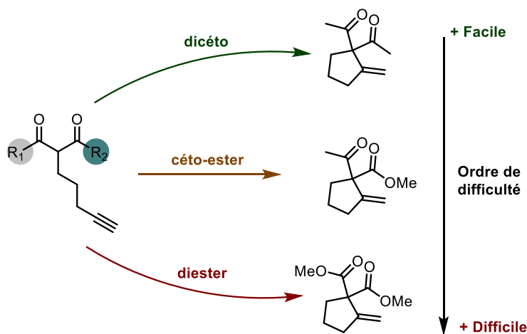
Figure 2: Ordre de difficulté de cyclisation de type Conia-ène des substrats dicéto, céto-esters et diesters
