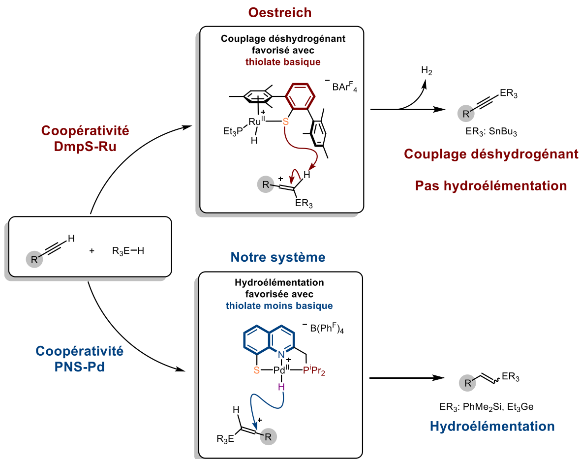
Schème 25: Comparaison des deux systèmes DmpS-Ru et PNS-Pd proposant une explication pour la différence de réactivité des deux systèmes
