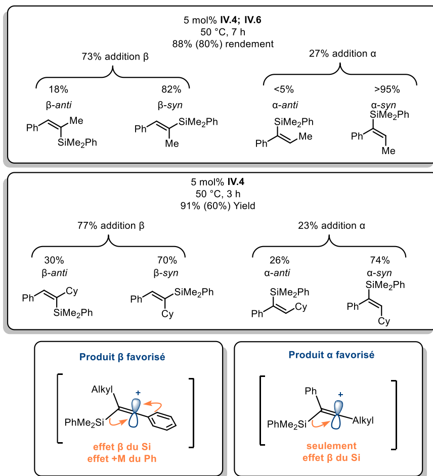
Scheme 22: Hydrosilylation catalytique d'alcynes dissymétriques Aryl-Alkyl
