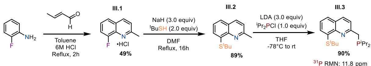
Scheme 6: Synthèse du ligand PNS en partant de la 2-fluoroaniline
