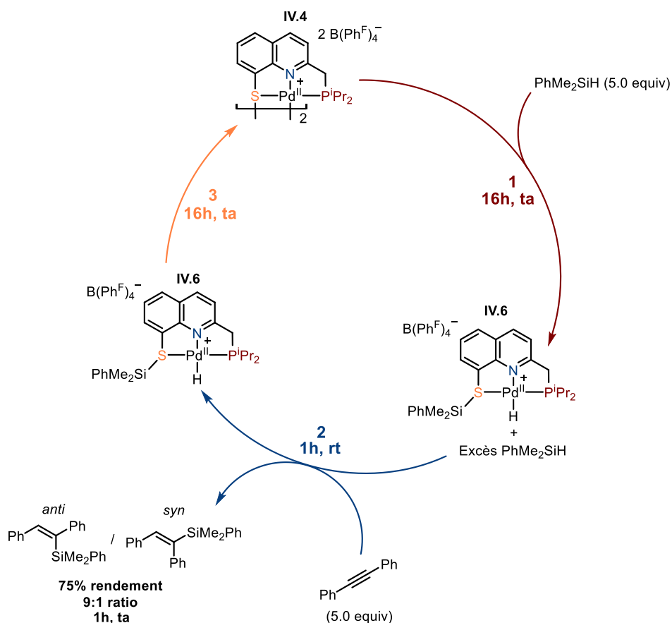
Scheme 18: Expériences de transferts Si-H "stœchiométriques"
