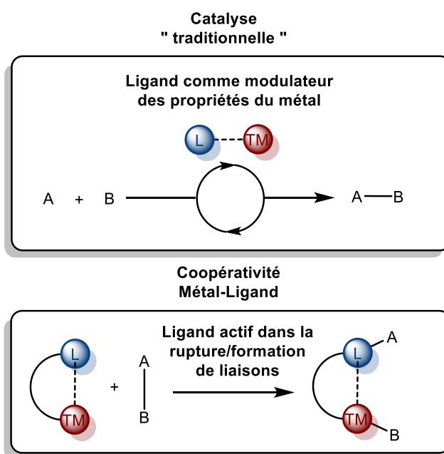
Scheme 1: Comparaison de la catalyse homogène traditionnelle et de la coopérativité métal-ligand
