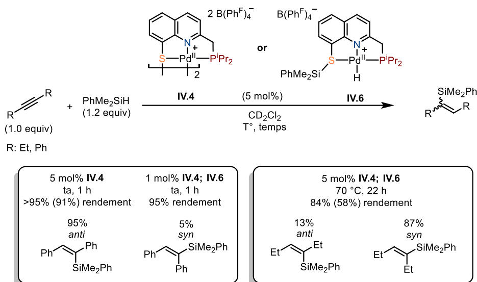
Scheme 19: Hydrosilylation catalytique d'alcynes internes symétriques
