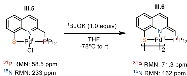
Scheme 9: Génération de l'espèce désaromatisée en présence d'une base
