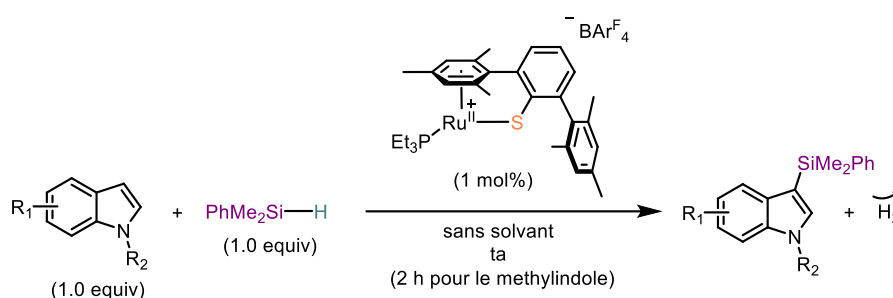
Scheme 15: Silylation déshydrogénante du méthylindole par le complexe DmpS-Ru
