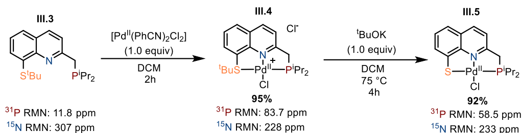
Scheme 7: Complexation du ligand PNS sur le palladium et formation de la plateforme III.5
