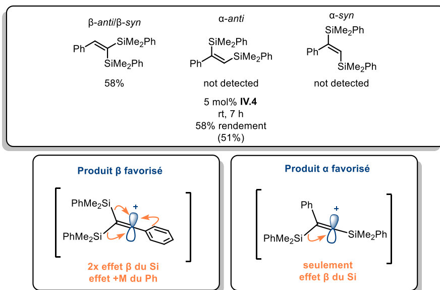
Scheme 2329: Hydrosilylation d'alcyne interne biaisé électroniquement et stabilisation des carbocations vinyliques correspondants
