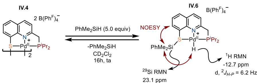
Scheme 17: Rupture hétérolytique de la liaison Si-H par le motif Pd-S
