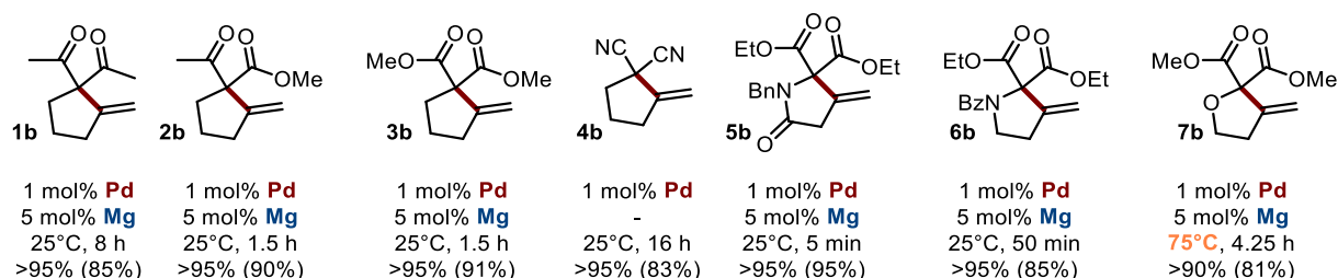
Figure 4: Produits de cyclisations 5-exo obtenus
