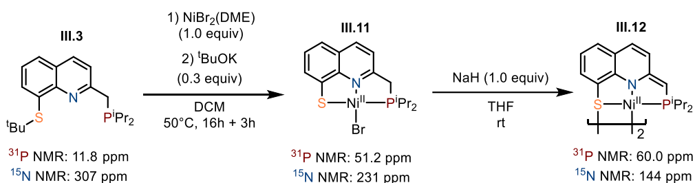
Scheme 14: Synthèse du complexe de PNS de nickel
