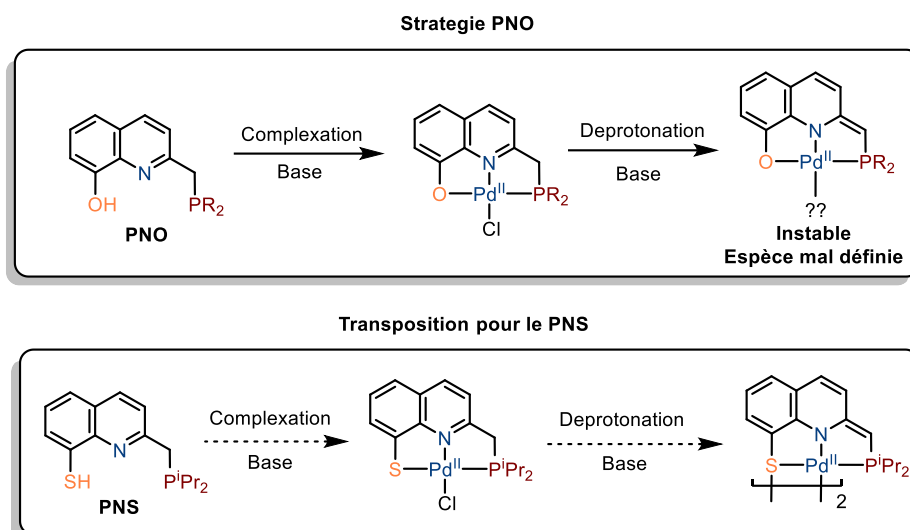
Scheme 5: Transposition de la synthèse développée pour le PNO avec la nouvelle architecture PNS et conséquences sur la formation d'une espèce binucléaire désaromatisée
