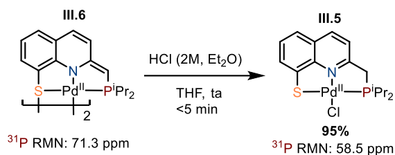
Scheme 10: Régénération du complexe neutre par traitement du complexe désaromatisé avec HCl
