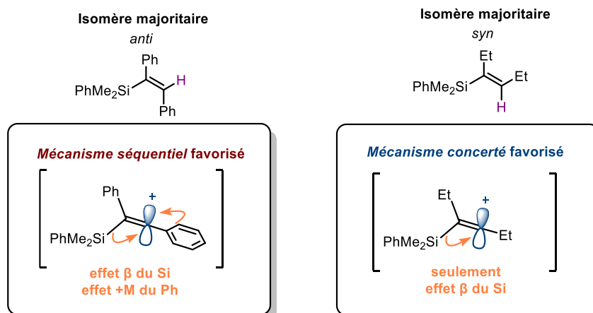
Scheme 21: Formation d'un carbocation vinylique dans le cas du tolane et de l'hex-3-yne et illustrations des effets stabilisants dans les deux cas
