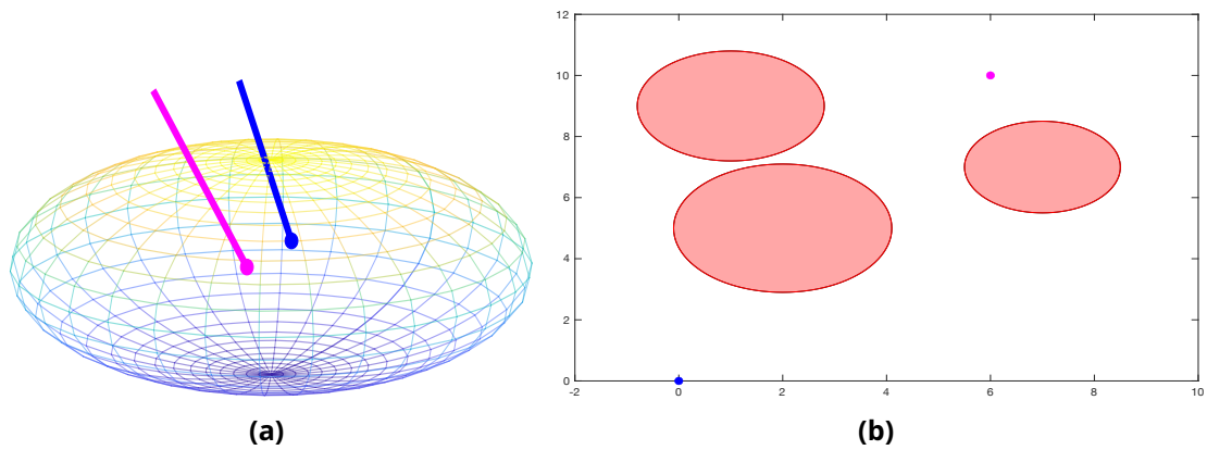
Figure A.9: Côté gauche: boule aplatie avec points de contact initiaux et finaux et ses orientations. Côté droit: obstacles (en rouge) et points de contact initiaux et finaux sur le plan.
