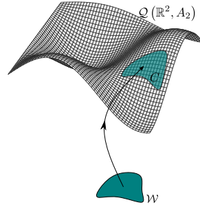
Figure A.4: Application d'obstacles dans M .
