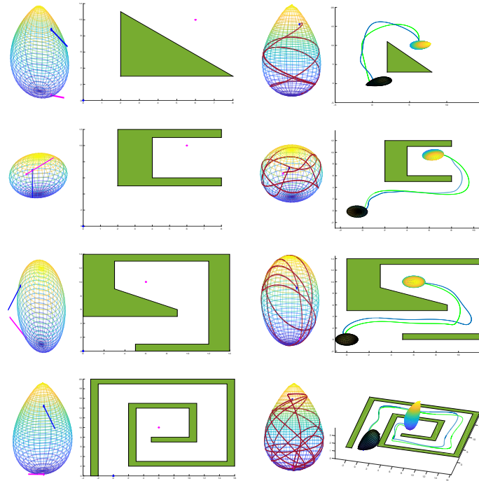
Figure A.11: Côté gauche: corps convexe avec points de contact initial et final avec orientations et obstacle sur le plan (en vert). Côté droit: courbe \gamma_2 sur le corps convexe et courbe obtenue en appliquant la méthode de continuation (en bleu) à la courbe initiale choisie (en vert).
