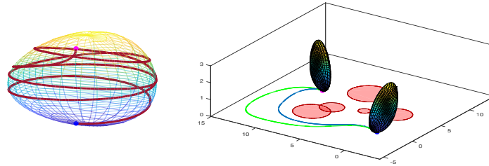
Figure A.12: Côté gauche: Corps convexe non symétrique avec points de contact initial et final et courbe \gamma_2 . Côté droit: Courbe obtenue en appliquant la méthode de continuation (bleu) à la courbe initiale choisie (vert).
