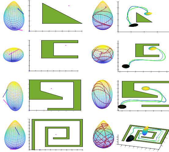
Figure A.2: Différents exemples de corps roulant sur le plan avec des obstacles.
