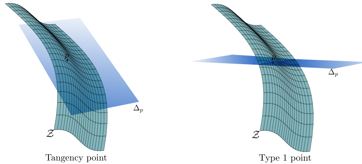
Figure A.1: Deux points différents forment \mathcal{Z} dans le cas générique 3D.
