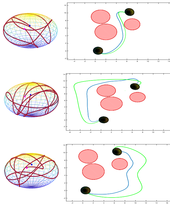
Figure A.10: À gauche: courbe \gamma_2 sur la boule aplatie. Côté droit : Courbe obtenue en appliquant la méthode de continuation (bleu) à la courbe initiale choisie (vert).
