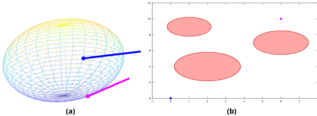
Figure A.5: Côté gauche: sphère avec points de contact initiaux et finaux et ses orientations. Côté droit : obstacles (en rouge) et points de contact initiaux et finaux sur le plan.
