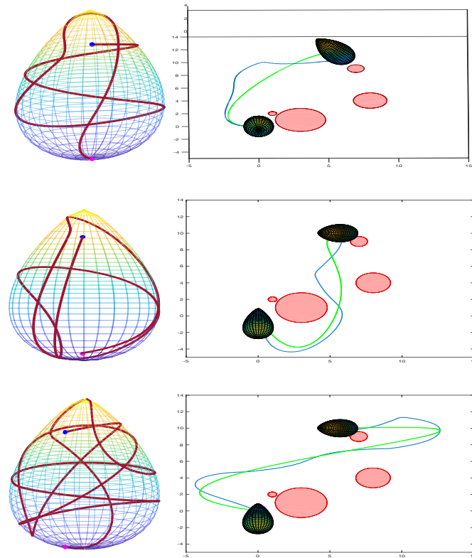
Figure A.8: À gauche: courbe \gamma_2 sur le oeuf. Côté droit : Courbe obtenue en appliquant la méthode de continuation (bleu) à la courbe initiale choisie (vert).
