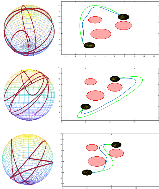
Figure A.6: À gauche: courbe \gamma_2 sur la sphère. Côté droit : Courbe obtenue en appliquant la méthode de continuation (bleu) à la courbe initiale choisie (vert).
