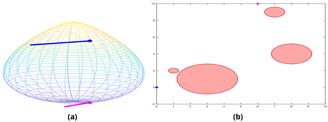
Figure A.7: Côté gauche: oeuf avec points de contact initiaux et finaux et ses orientations. Côté droit: obstacles (en rouge) et points de contact initiaux et finaux sur le plan.
