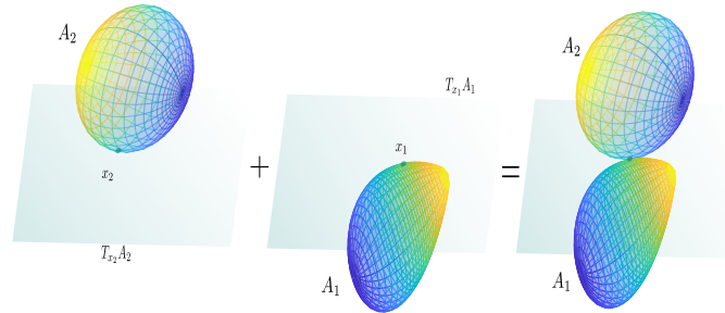
Figure A.3: Idétification des espaces tangents au point de contact.
