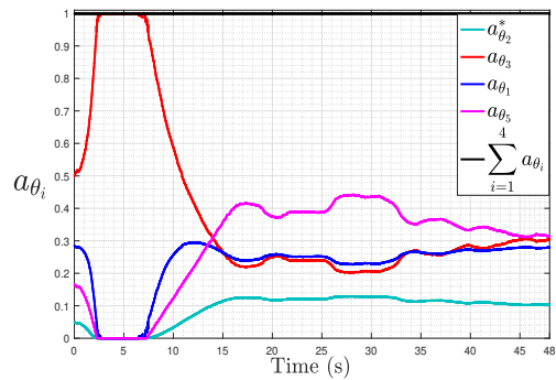
(d) Real-time solution of the LS (4.23), a_{\theta_i}
