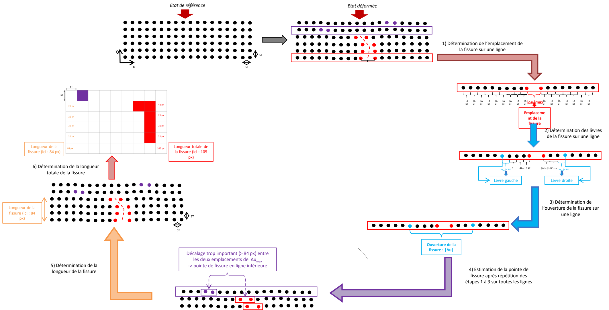
Figure II.16 : Schéma de l'étude du processus de fissuration en flexion
