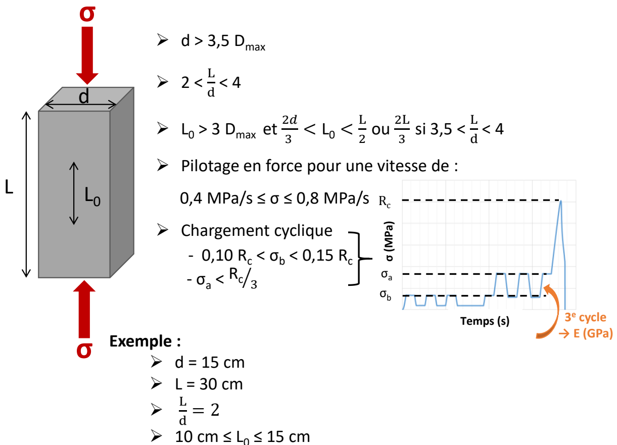
Figure IV.7 : Exigences de la norme NF EN 12390-13 [190] pour le calcul du module d'élasticité sécant des bétons
