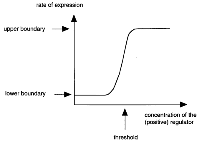
FIGURE 1.2 – Évolution sigmoïdale du taux d'expression d'une molécule en fonction de la concentration d'un régulateur. Schéma tiré de (THOMAS et al., 1995).
