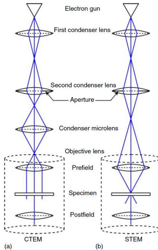
Figure III.8 : Schémas des configurations des lentilles dans la partie supérieure du microscope électronique et leurs influences sur les trajectoires du faisceau d'électrons pour CTEM (a) et STEM (b). Reproduit avec permission [71]. Copyright 2016, Wiley-VCH.
