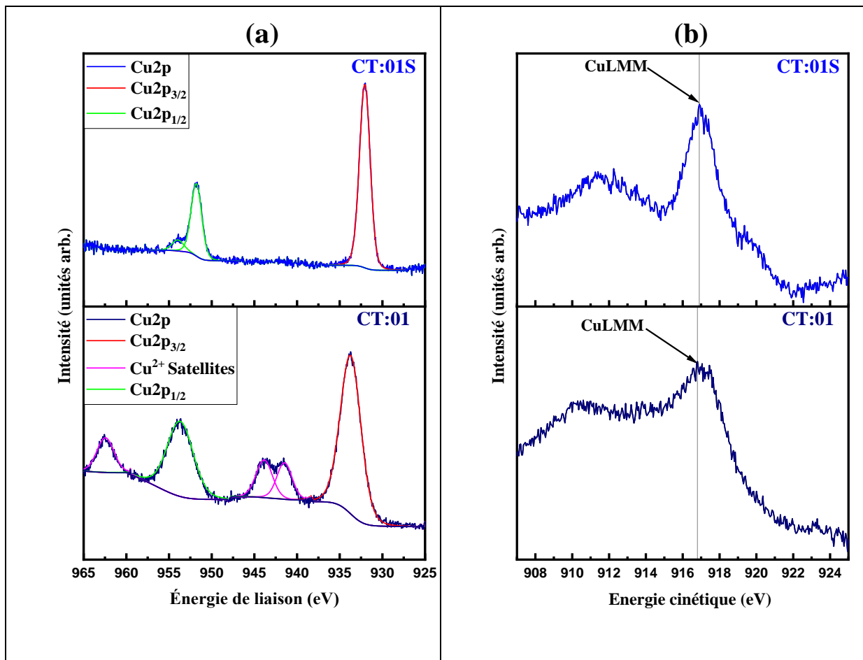
Figure IV.6 : Niveaux de cœur XPS et position de Auger du cuivre pour les échantillons CT:01 et CT:01S.
