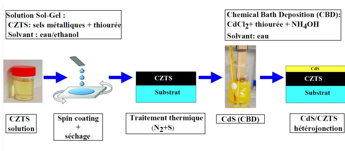
Figure V.1 : Schéma du procédé de fabrication de l'hétérojonction CdS/CZTS.
