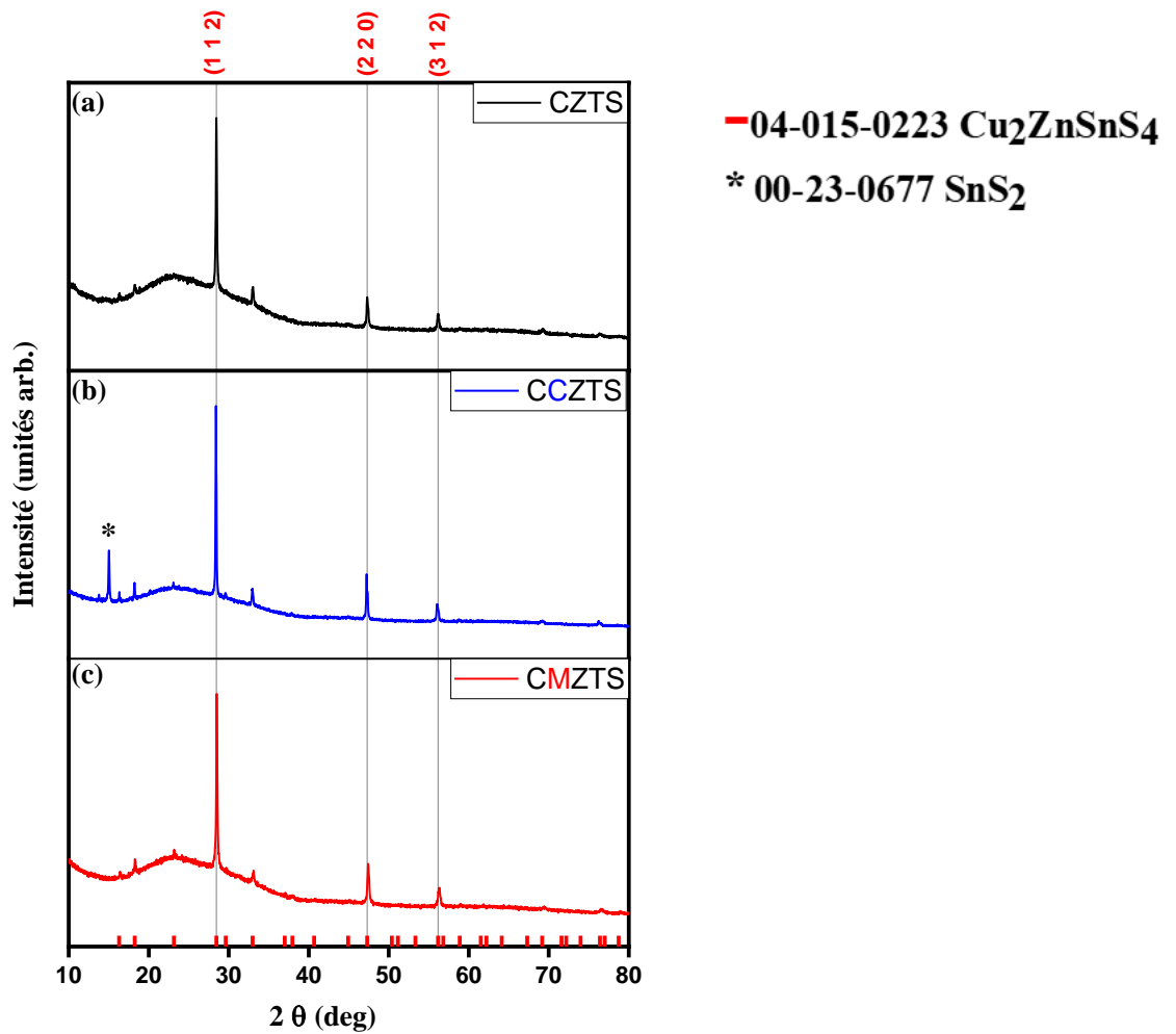
Figure VI.2 : Diffractogramme des rayons X des échantillons CZTS, CCZTS et CMZTS.
