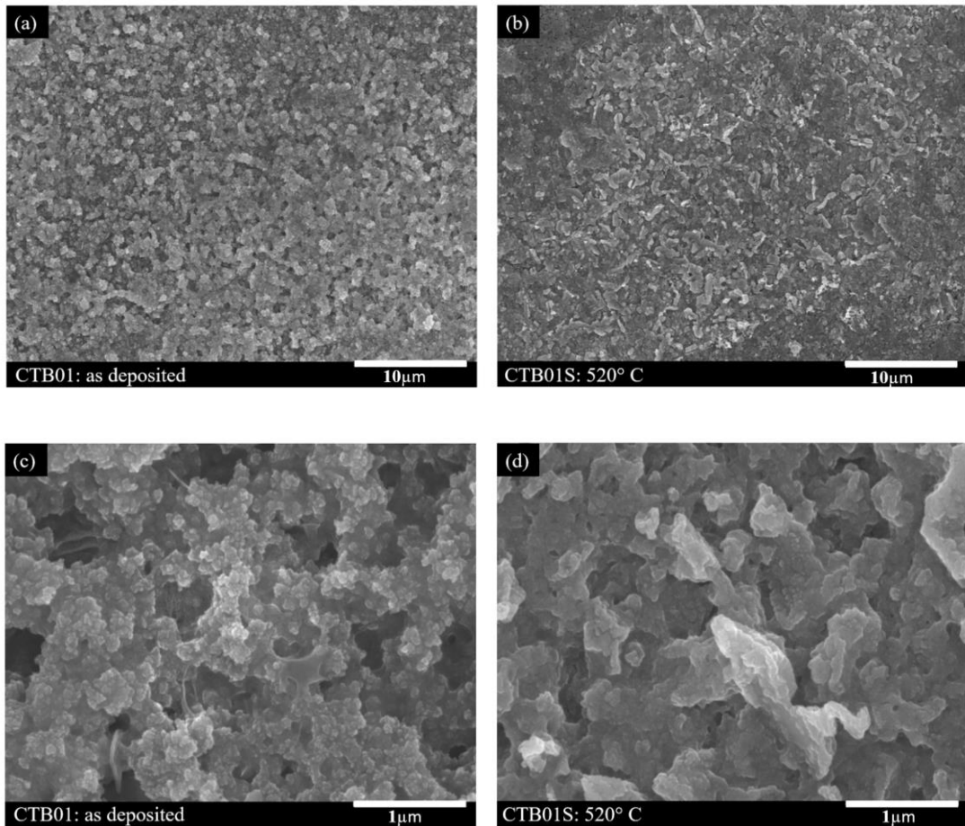
Figure IV.19 : Images SEM des couches minces du CZTS. (a-c) avant traitement thermique CTB01, (b-d) après traitement thermique de l'échantillon CT :B01S.
