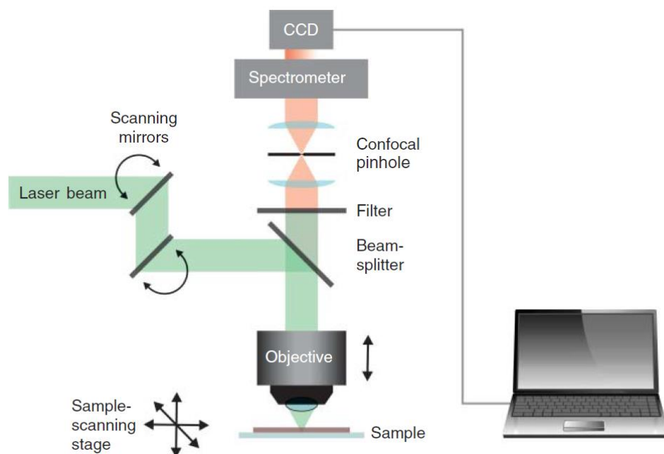
Figure III.6 : Montage d'une spectroscopie Raman couplée à un microscope optique.
