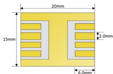
Figure VII.2 : Conception du substrat ITO à 8 pixels fourni par Ossila [142].
