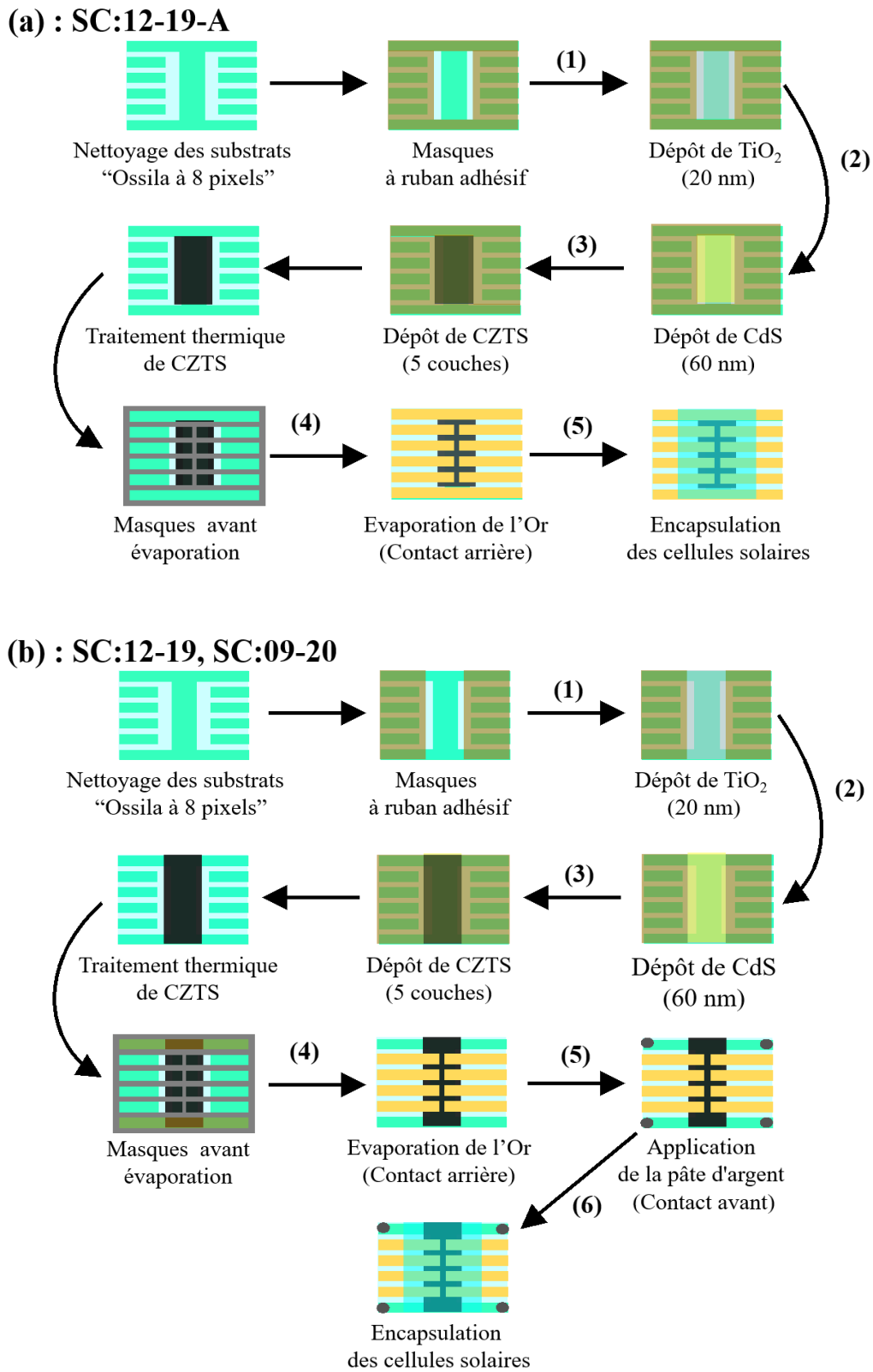
Figure VII.3 : Les différentes étapes suivies pour la fabrication de cellules solaires en couches minces de type CZTS en configuration superstrat.
