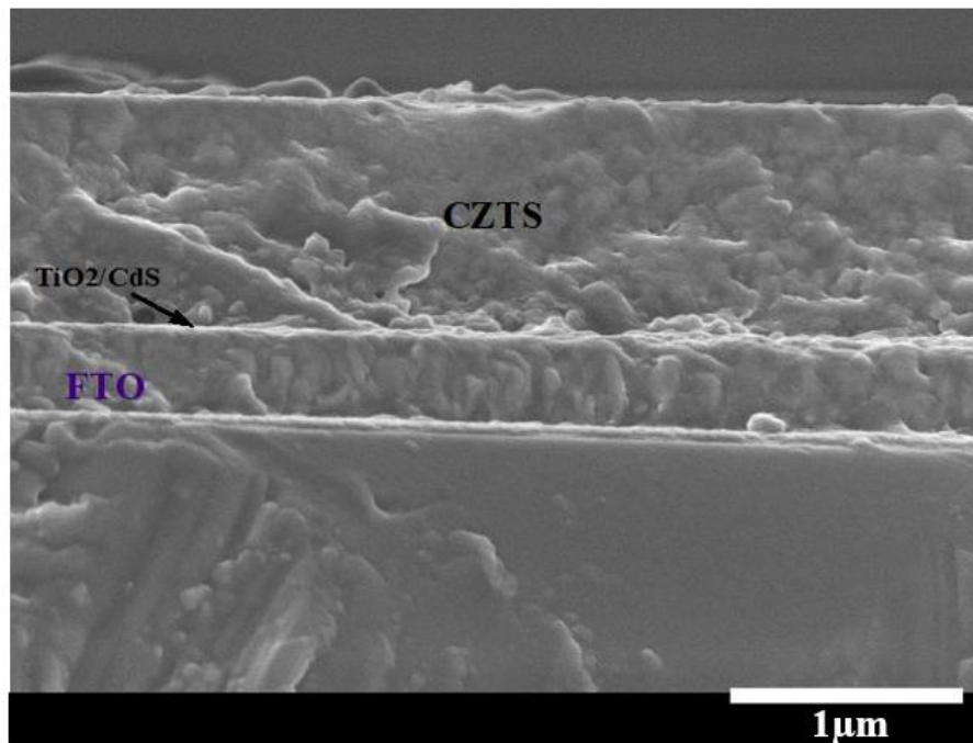
Figure VII .15 : Micrographie SEM en coupe transversale de la cellule solaire SC:20-01.
