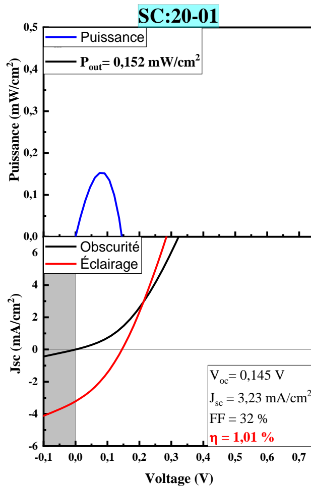
Figure VII .11 : Courbes J-V et P-V de la cellule solaire SC :20-01.
