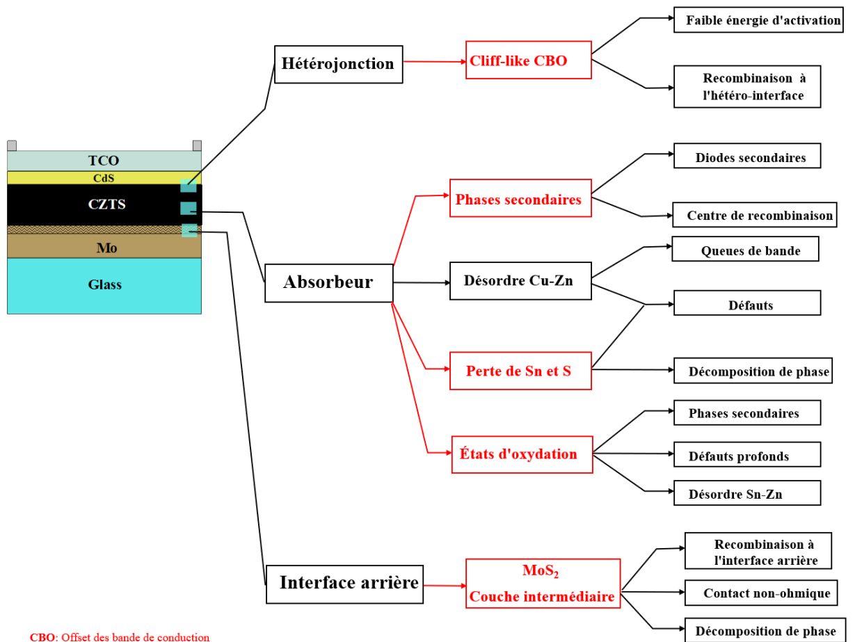
Figure II.6 : Les principaux problèmes limitant l'efficacité des cellules solaires CZTS.
