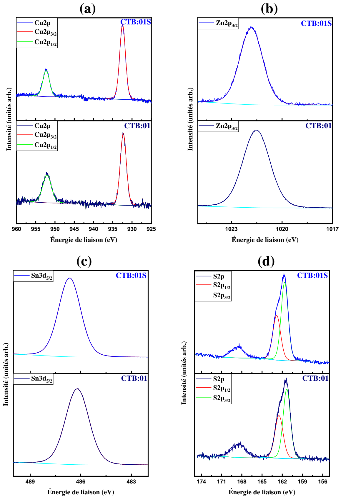
Figure IV.18 : Spectres XPS des couches minces du CZTS avant et après le traitement thermique. (a) Cu2p (b) Zn2p 3/2 (c) Sn3d 5/2 et (d) S2p.
