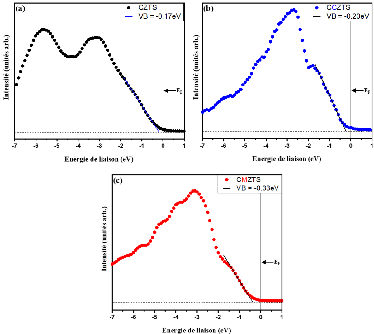
Figure VI.6 : Estimation de la position de la bande de valence à partir des mesures XPS. (a) CZTS, (b) CCZTS, (c) CMZTS .
