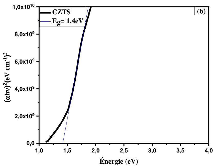
Figure V.5 : La bande interdite optique obtenue à partir de mesures dans l'UV/Visible (a) CZTS, (b) CdS.
