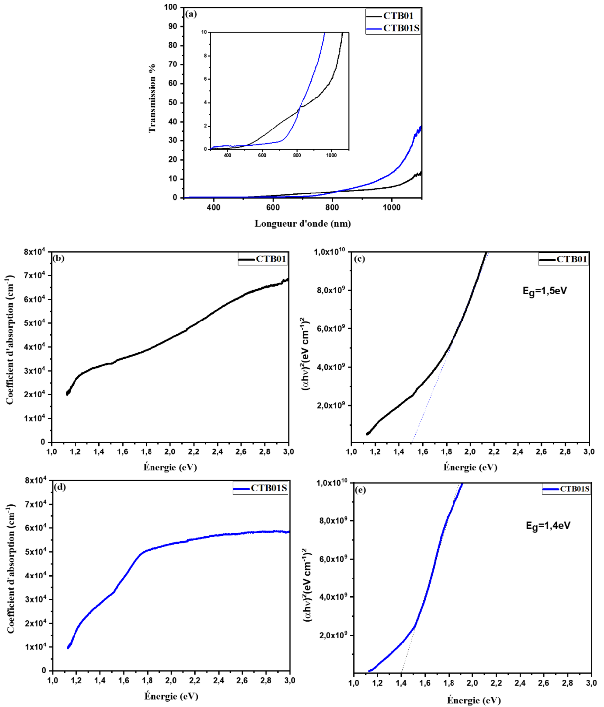
Figure IV.20 : (a) Transmittance des couches minces CZTS ; Coefficient d'absorption des couches minces CZTS en fonction de l'énergie (b) échantillon avant traitement thermique CTB01 (c) échantillon après traitement thermique CT:B01S ; Bande interdite des couches minces CZTS (d) CT:B01 (e) CT:B01S
