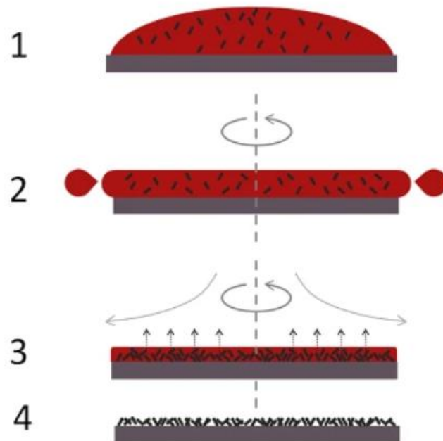
Figure III.1 : Les différentes étapes de la technique de dépôt par spin coating [67].
