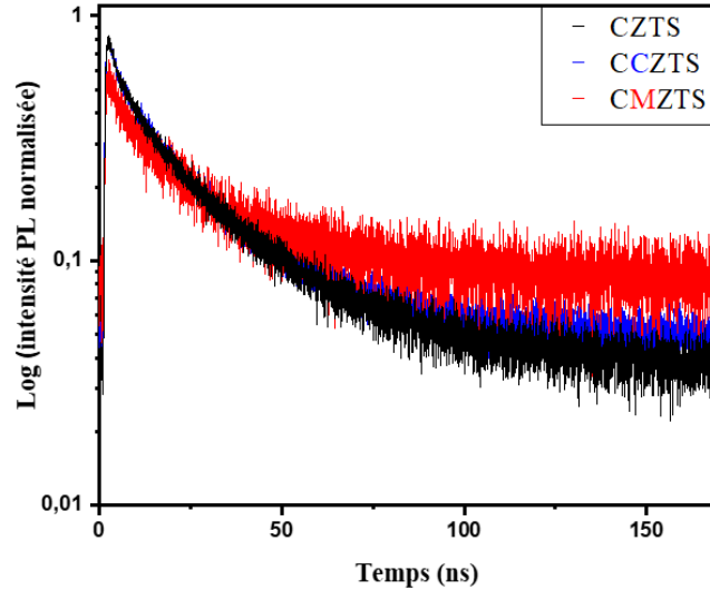
Figure VI.11 : Décroissance de la photoluminescence normalisée et résolue en fonction du temps avec une longueur d'onde d'excitation de 488 nm. Couleur noire CZTS/CdS, couleur bleue CCZTS/CdS et couleur rouge CMZTS/CdS.
