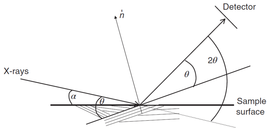
Figure III.4 : Représentation schématique de l'expérience de DRX en incidence rasante : \alpha est l'angle d'incidence, \theta l'angle de Bragg et n la normale du plan du réseau qui répond à la loi fondamentale de Bragg. Reproduit avec permission [68]. Copyright 2016, Wiley-VCH.
