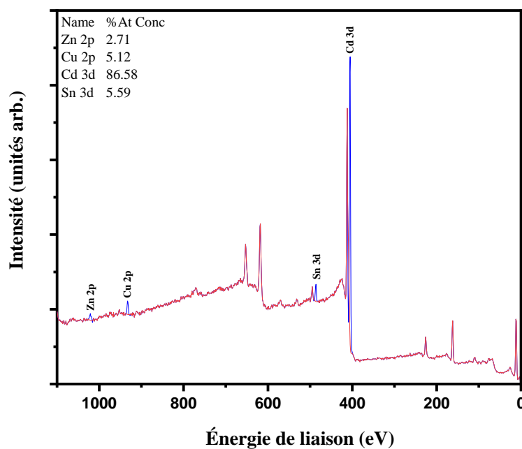
Figure V.3 : Spectre d'analyse chimique XPS après 180 secondes de pulvérisation..
