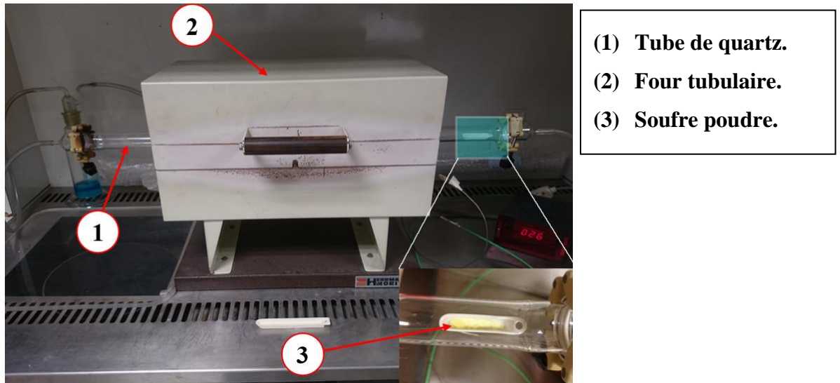
Figure IV.2 : Montage employé pour l'incorporation de soufre (" PSC ").
