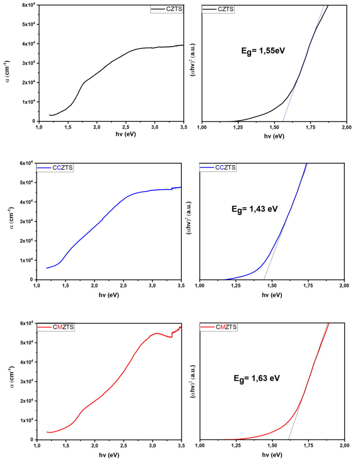
Figure VI.5 : Estimation de l'énergie de gap et du coefficient d'absorption à partir des mesures UV/Visible. (a) CZTS, (b) CCZTS, (c) CMZTS.
