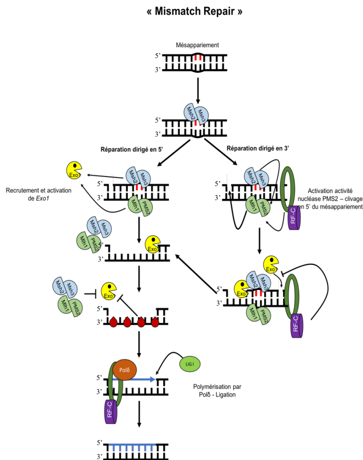
Figure 7 : Schéma des différents mécanismes de réparation par le « Mismatch repair ». La reconnaissance des mésappariements est réalisée par le complexe MSH2-MSH6/MSH3 (MutSα et MutSβ respectivement). La réparation d'un mismatch nécessite la présence d'un gap en 5' ou 3' de la lésion. Une réparation dépendante d'un gap en 5' ne nécessite pas l'activité nucléase de PMS2 du complexe MutLα. MutSα et MutLα vont stimuler l'activité exonucléase d' EXO1 qui digère le fragment portant la lésion. Lorsque MutSα et MutLα sont retirés de l'ADN, ils inhibent l'activité d' EXO1 conjointement avec RPA qui se fixe sur le fragment simple brin. Lors d'une réparation dépendante d'un gap en 3' de la lésion, MutLα, dont l'activité nucléase est stimulée par PCNA et MutSα, va induire une cassure simple brin en 5' de la lésion permettant à EXO1 de digérer le fragment portant la lésion. La réparation est terminée par la synthèse d'un nouveau fragment par l'ADN Polδ et l'ADN ligase I qui comble le gap.
