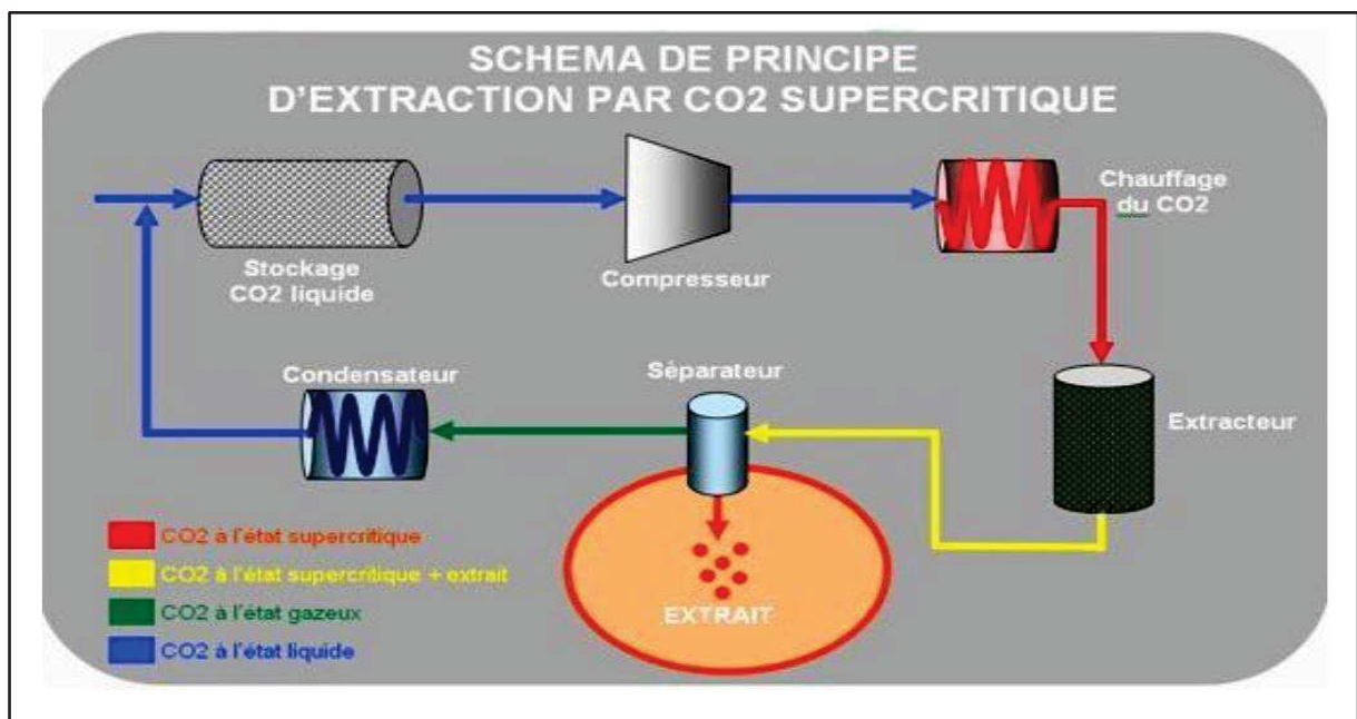
Figure 8 : Principe d'extraction par CO 2 supercritique ( http://www.biostimulants.fr/wp-content/uploads/2019/02/schema-1024x576.jpg ).
