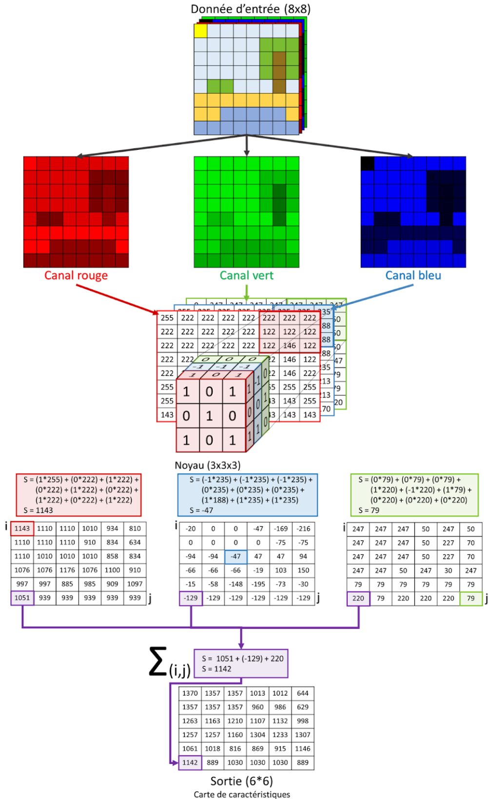
Figure 42 - Fonctionnement du processus de convolution sur une image en couleur. La première étape consiste à scinder la donnée initiale en 3 canaux, un pour chaque couleur RVB. Chaque noyau est ensuite appliqué sur les différents canaux afin d'obtenir des cartes de caractéristiques temporaires. Les valeurs des éléments (i,j) sont sommées pour finalement obtenir la valeur (i,j) de la carte de caractéristiques.
