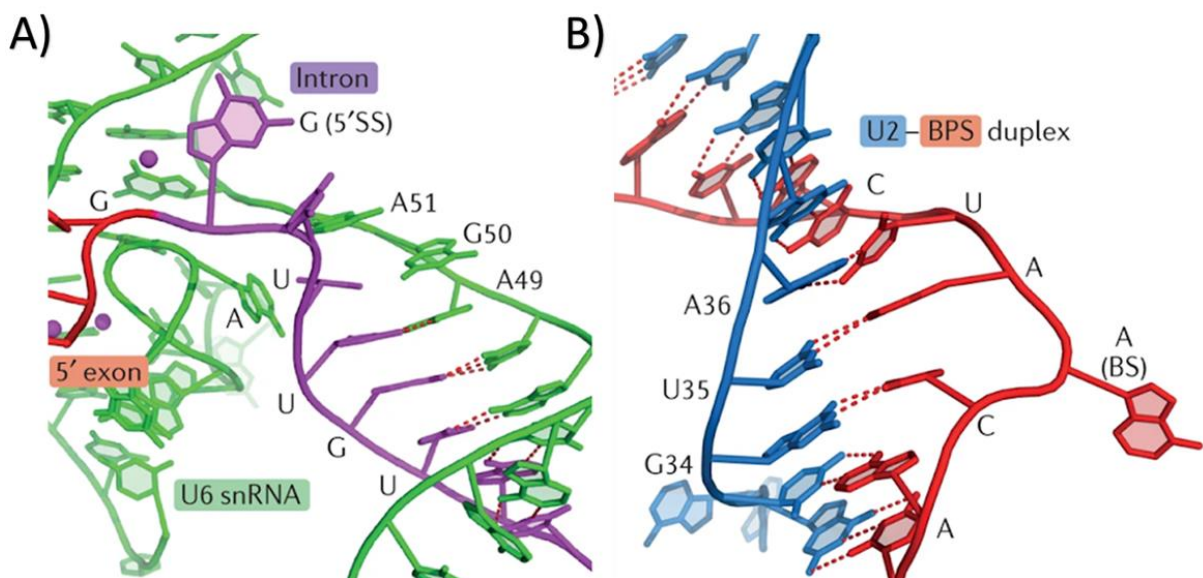
Figure 31 - Identification des éléments propices au déclenchement du mécanisme d'épissage par des snRNA du spliceosome. A) Reconnaissance du SE donneur (5'), les nucléotides UGU introniques s'apparient avec les nucléotides de la sous-unité snRNA U6. B) Formation de duplex entre la séquence de point de branchement (BPS) et la sous-unité snRNA U2 chez la levure (source : (Shi, 2017)).
