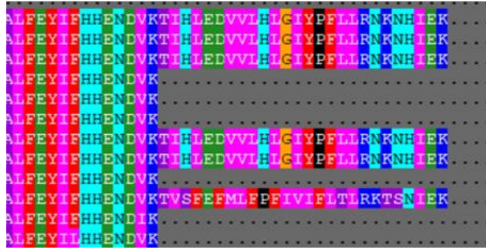
Figure 47 - Identification d'isoformes. Dans certains cas, il y a une séquence supplémentaire et dans d'autres elle est absente. Il ne s'agit pas d'une insertion ou d'une délétion provoquée par une erreur, mais bien d'une isoforme, car des espèces proches présentent également ce même fragment.
