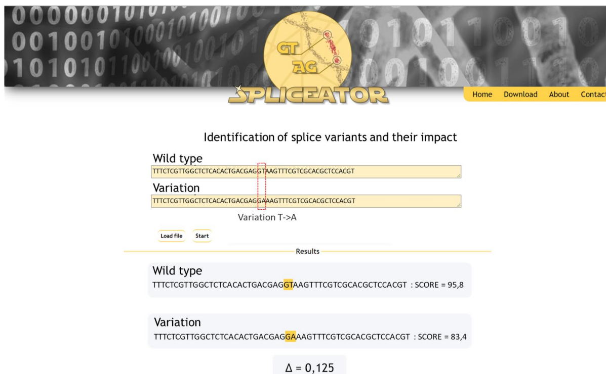
Figure 61 - Maquette de la mise à jour du site web de Spliceator pour la prédiction de variants d'épissage. Deux séquences sont comparées (wild type vs disease causing) afin d'évaluer l'impact d'une variation.
