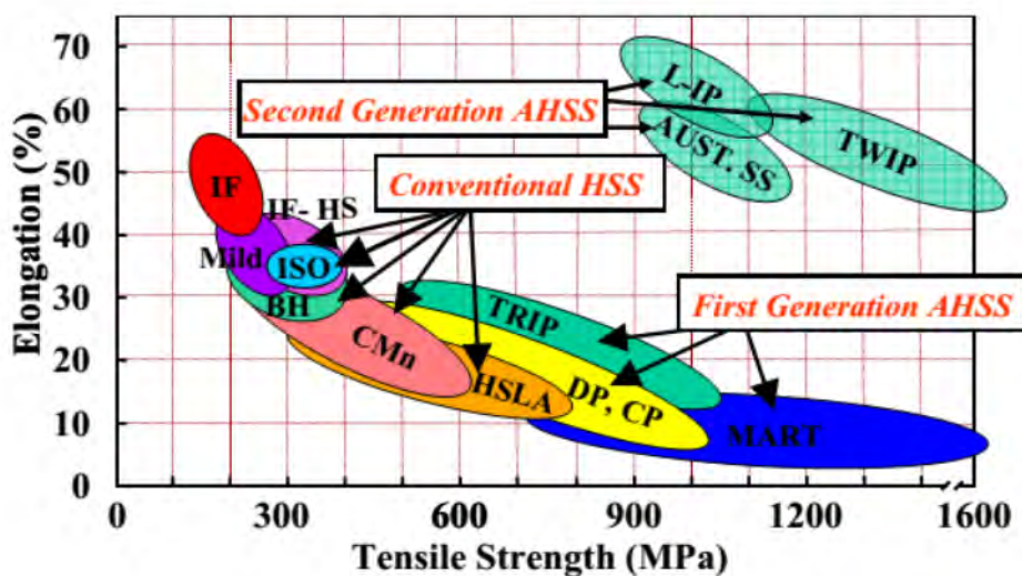
FIGURE 1.7 – Diagramme élancement en fonction de la résistance mécanique pour différents types d'aciers [18]
