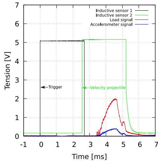
FIGURE 4.4 – Signaux mesurés durant l’essai grâce aux différents capteurs
