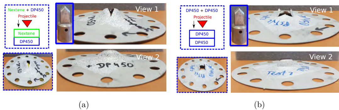
FIGURE 4.14 – Structures impactées avec le cap diédrique. (a) Nextene + DP450. (b) DP450 + DP450
