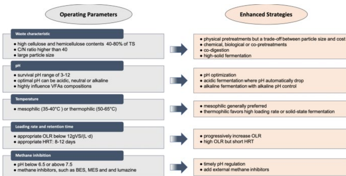
Figure I-17 : Résumé des optimisations possibles des paramètres de la digestion anaérobie pour la production d'acides gras volatils. D'après Sun et al., (2021).
