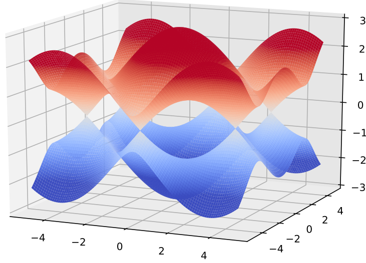
FIGURE 1.2 – Le modèle de Wallace. La relation de dispersion est invariante par rotation de \pi/3 autour de l'origine. On observe des points de Dirac à l'intersection entre les deux bandes.
