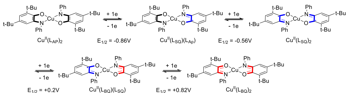
Schéma R-8. Propriétés redox de Cu(L SQ ) 2
