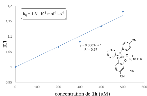
Figure R-5. Tracé de Stern-Volmer - extinction du silicate 1h et 3 . Ce travail a été réalisé par le Dr. Etienne Levernier.
