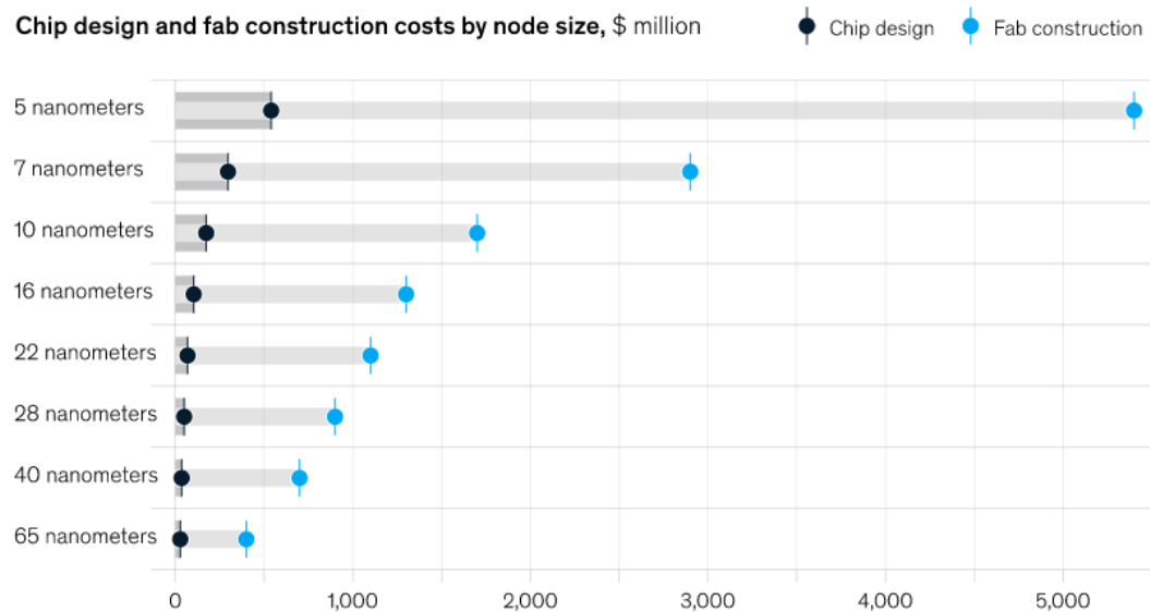
FIGURE 1.8 – Coût du design et de la fabrication de puce électronique en fonction de la taille des noeuds (source : McKinsey & Company, IBS : McKinsey analysis)
