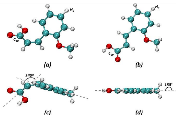
图 2.5 使用 M052X/6-31G* 基组优化后的 trans/cis -OMCA 分子结构。
