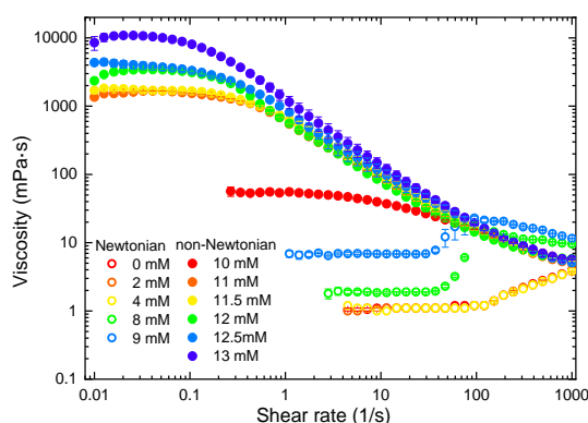
图 5.1 20 mM CTAB 和 0-13 mM NaSal 溶液在 22°C 时的流动曲线。
