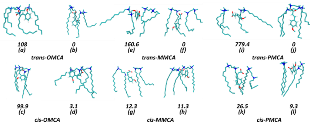
图 4.6 12-3-12 2+ 和 OMCA、MMCA、PMCA 在胶束上不同排布方式和相应的相互作用能 (kJ/mol)。在(a)、(d)、(e)、(h)、(i)、(l)中, 苯环分布在胶束表面。在(b)、(c)、(f)中, (g)、(j)、(k)中, 苯环嵌入 12-3-12 2+ 的烷基链中。为清楚起见, 未显示和甲氧基和 12-3-12 2+ 上的氢原子。为方便起见, 将苯环嵌入胶束中的反式异构体排布方式的相互作用能设为 0 kJ/mol。)
