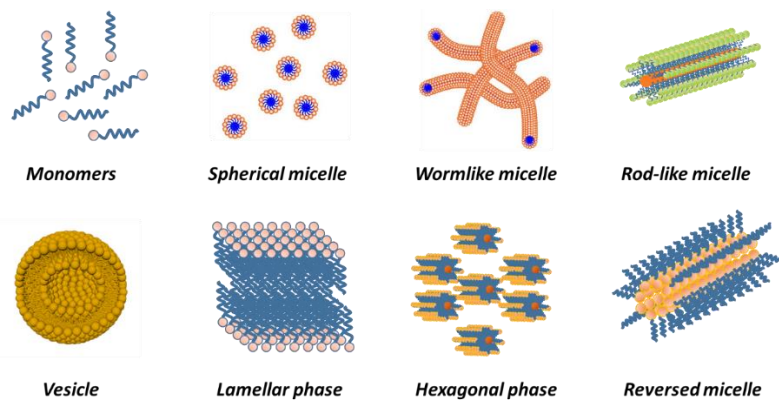
图 1.1 常见的表面活性剂自组装体种类
