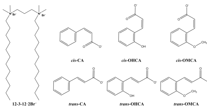
图 3.1 Gemini 表面活性剂 12-3-12·2Br - 和肉桂酸衍生物 cis/trans -CA、 cis/trans -OHCA 和 cis/trans -OMCA 的分子结构
