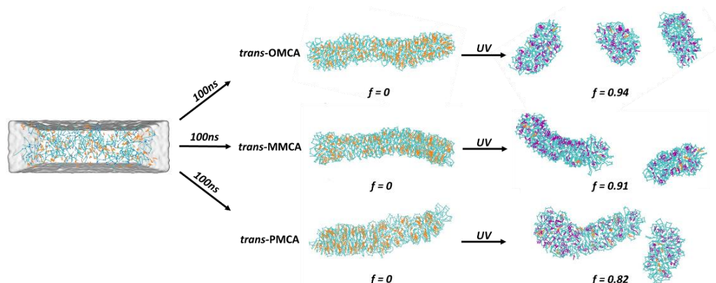
图 4.2 25℃下 180 个 12-3-12 2+ 和 135 个 trans -OMCA, trans -MMCA, trans -PMCA 混合体系初始构型和在平衡转化率下经过 100 ns 分子动力学模拟后的最终构型的快照。(青色部分为 12-3-12 2+ ；橙色部分为反式异构体；红色部分为顺式异构体。为清楚起见，水、Br - 和 Na + 未显示。)
