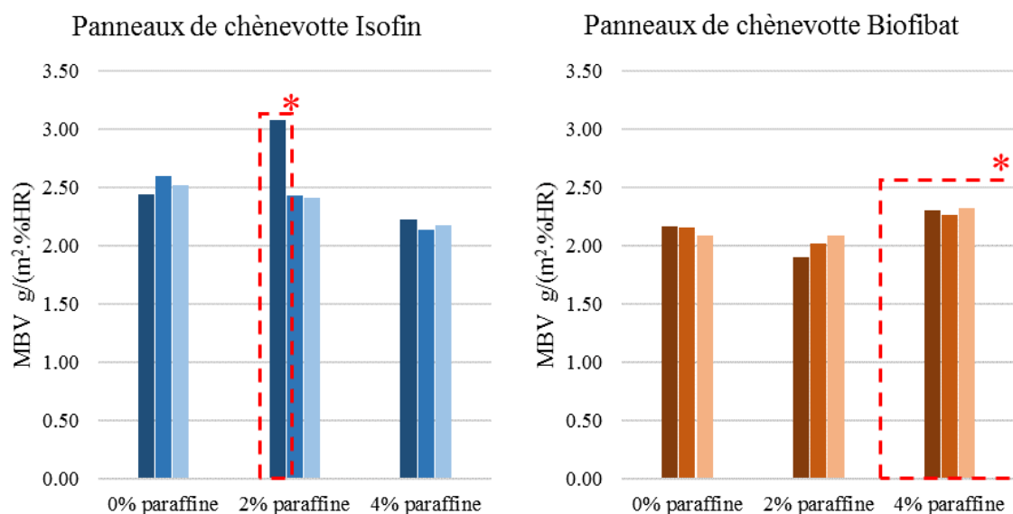
Figure IV-24: Effet de la paraffine et de la taille des granules de chènevotte sur le MBV
