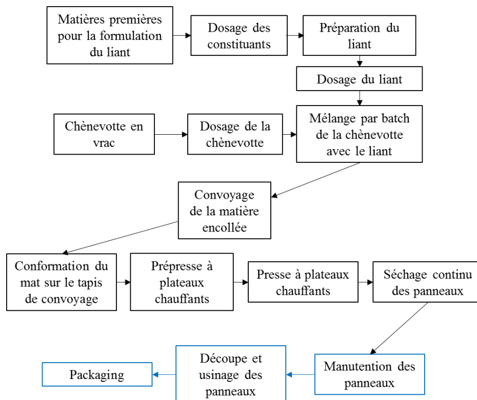
Figure V-18 : Schéma des étapes de fabrication de la ligne de production testée
