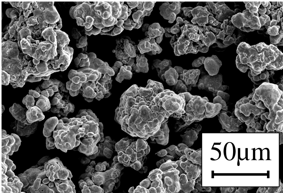
Fig. 2-1 SEM image of pure Cu powder.
