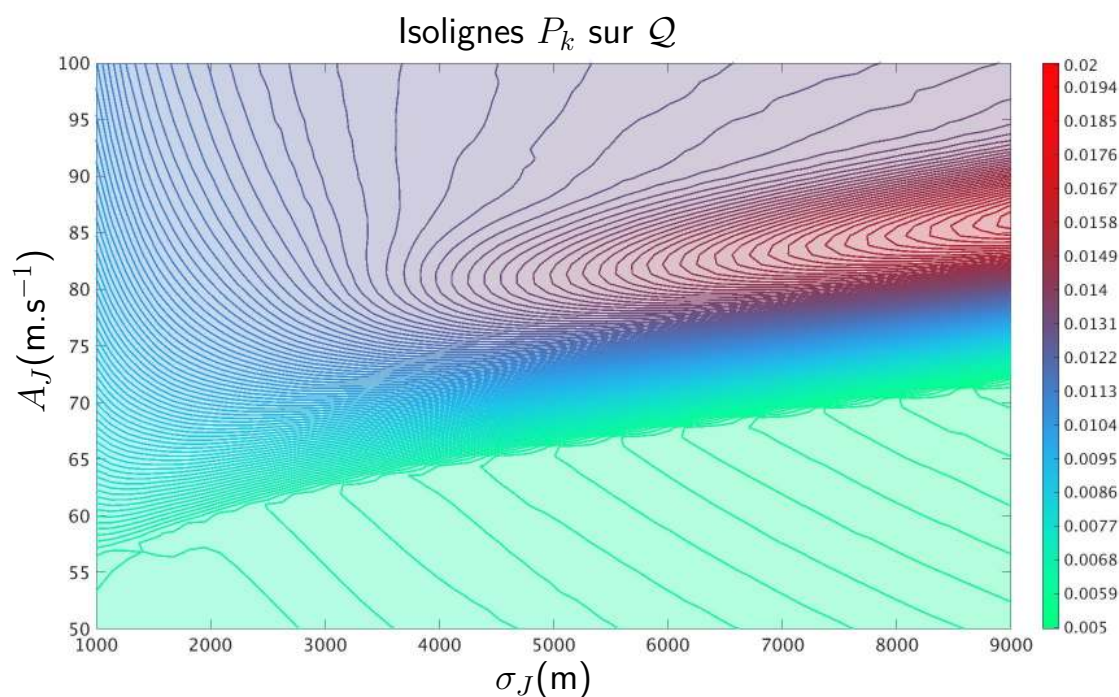
Figure 4.11 : Amplitude maximale P_k des signaux enregistrés à 285 km de la source en fonction des paramètres de jet stratosphérique A_J et \sigma_J . Les iso-valeurs vont de 5.0 \times 10^{-3} Pa à 2.0 \times 10^{-2} Pa.
