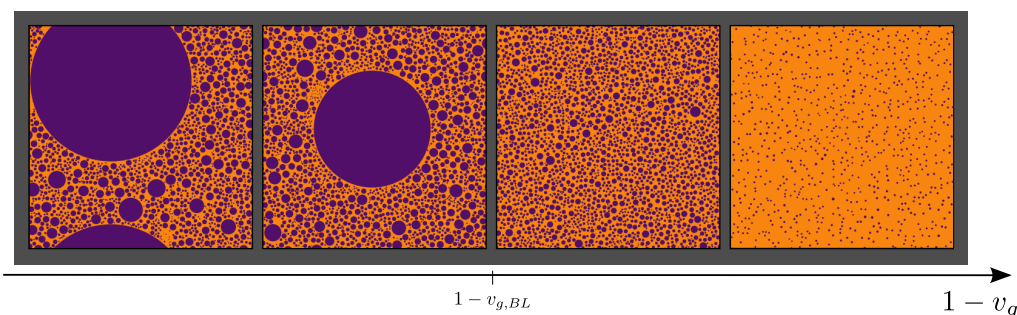
Figure 6.5: Diagramme de phase de taille finie à faible diffusivité. Nous pouvons observer l'émergence d'un état de micro-séparation de phase que nous identifions avec le liquide bouillonnant, et un état de macro-séparation de phase entre une grande bulle et une mer de bulles plus petites autour (séparation de phase bouillonnante). De gauche à droite, les fractions de vapeur diminuent (donc la densité globale \phi_0 augmente).
