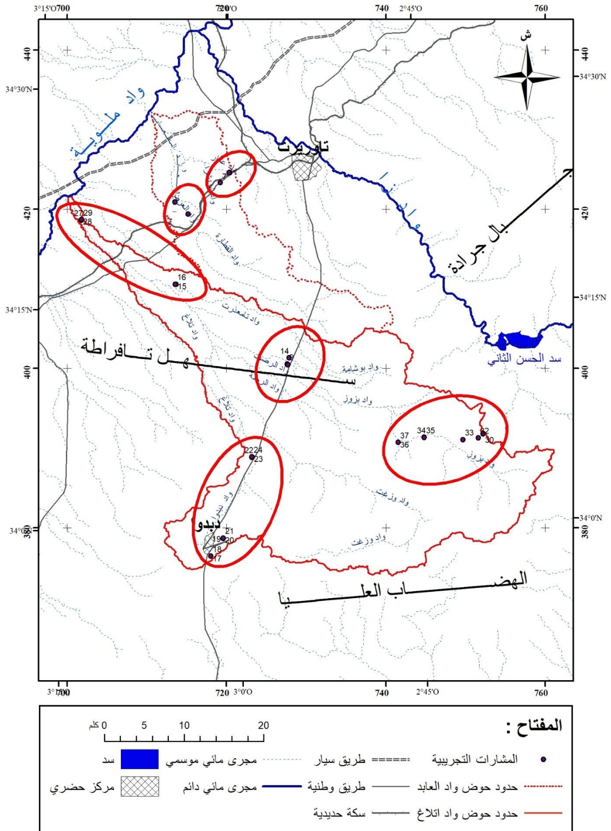
الشكل رقم 61: توطين المشارات التجريبية
