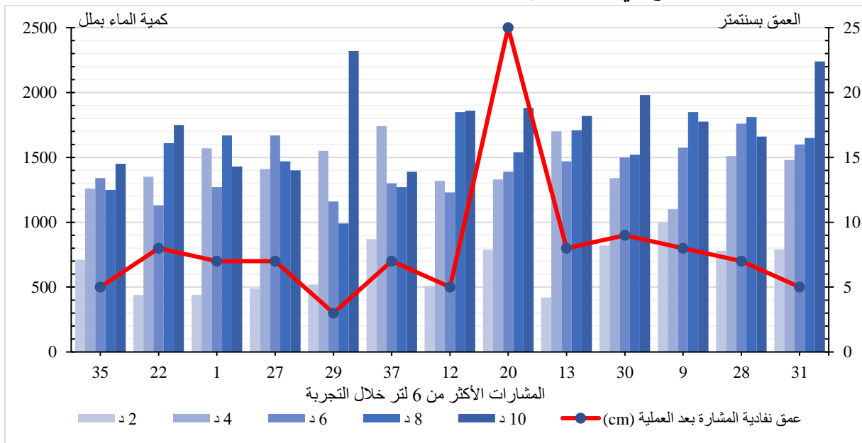
الشكل رقم 71: تطور الحجم الإجمالي للسيلان بالمشاركات التجريبية الأكثر من 6 لتر.
