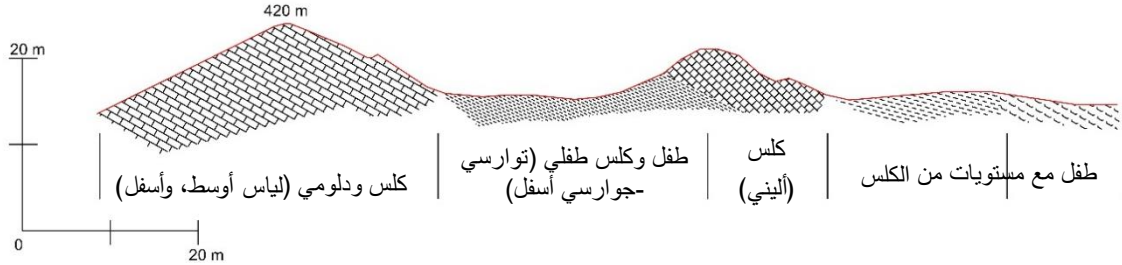
الشكل رقم 119: مقطع جيولوجي من الكدية الزرقة إلى وادي العابد قرب حامة سيدي شافي
