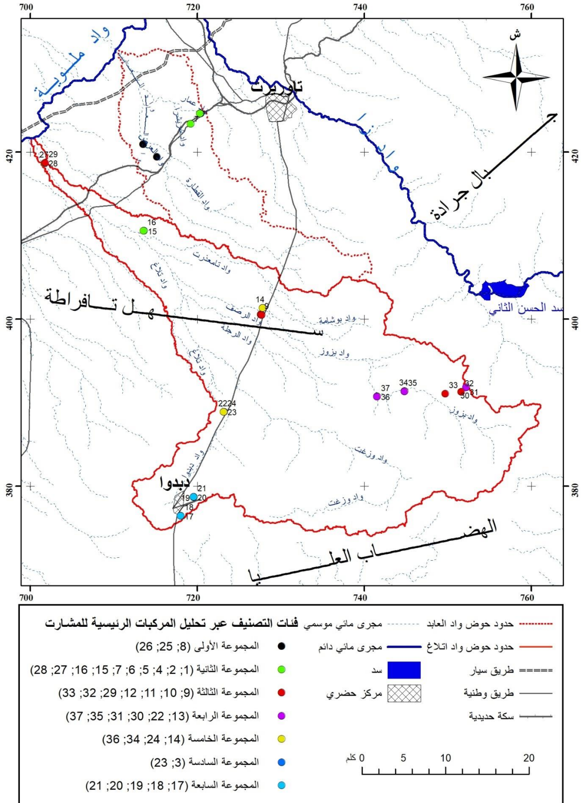
الشكل رقم 85: فئات التصنيف عبر تحليل المركبات الرئيسية للمشارت التجريبية
