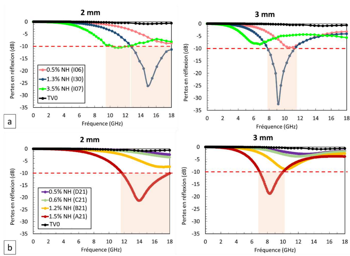
Figure IV.4 – Courbes de pertes en réflexion des composites NTC-TV/époxy à morphologie inhomogène pour des épaisseurs simulées de 2 mm et 3 mm. (a) tissus de synthèses CVD avec injection catalytique transversale et (b) tissus de synthèse CVD avec injection axiale
