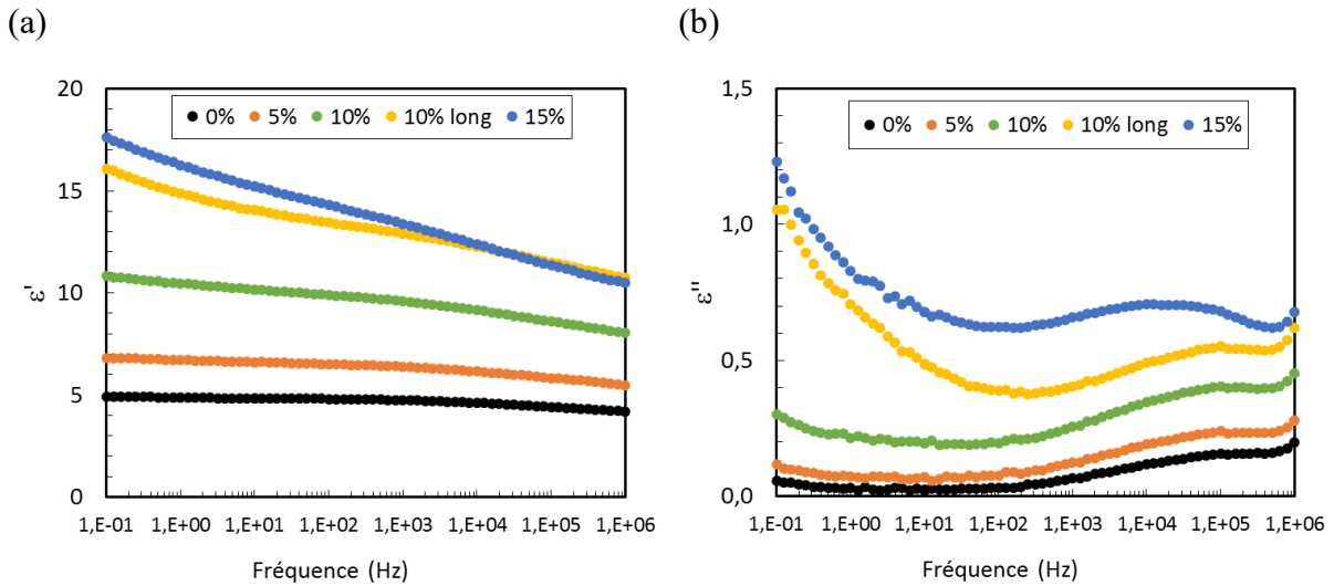
Figure III.23 – Parties (a) réelle et (b) imaginaire de la permittivité des composites NTC Timesnano /époxy jusqu'à 1 MHz. L'échelle des ordonnées est volontairement différente pour plus de lisibilité.
