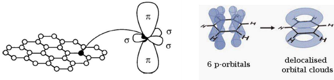
Figure I.19 – Orbitales \sigma et \pi du carbone en hybridation sp^2 dans un réseau hexagonal.
