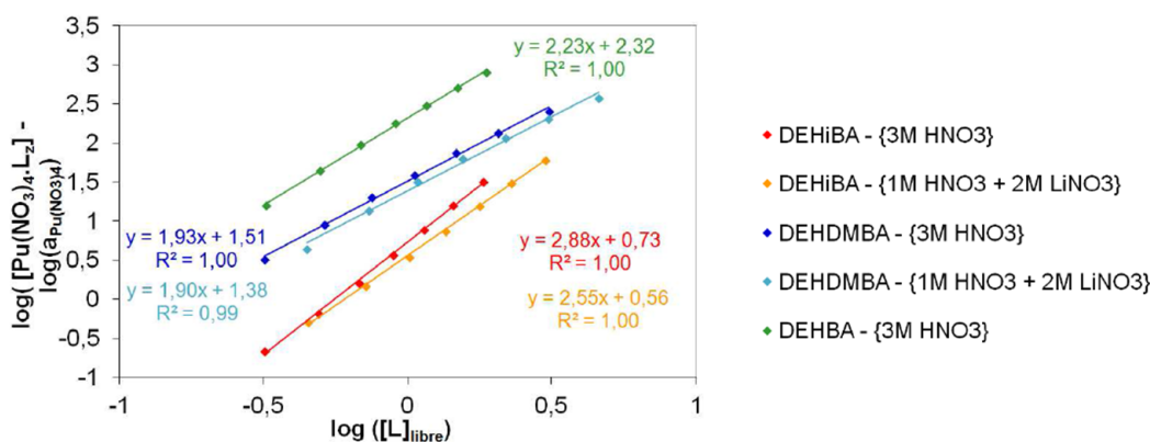
FIGURE 8 – Extraction du nitrate de plutonium par des solutions de DEHBA, DEHDMBA, DEHiBA en fonction de la concentration en extractant. Hypothèse retenue pour l'extraction d'acide nitrique : \{L(HNO_3), L_2(HNO_3), L(HNO_3)_2\} . Phase aqueuse : \{Pu(NO_3)_4 \cdot 10^{-4} \text{ mol.L}^{-1} + HNO_3\} . Phase organique : solution de dialkylamide dans le dodécane pré-équilibrée. Figure reproduite du travail de F. Rodrigues [22].
