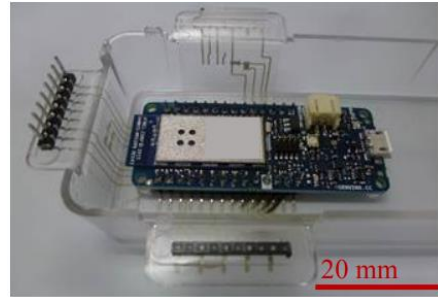
Figure I-32 : Boîtier intelligent réalisé en électronique moulée [18] a) vue de dessous b) vue de dessus
