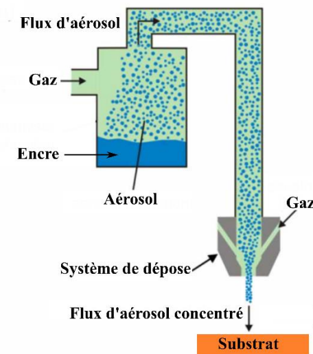
Figure I-13 : Principe de la technique de l'aérosoljet adapté de [75]
