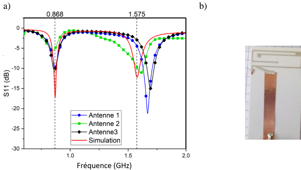
Figure III-46 : a) Mesure du paramètre S_{11} sur 3 antennes imprimées sur du plastique PC+ABS et simulation b) Photographie d'une antenne imprimée sur du plastique PC+ABS
