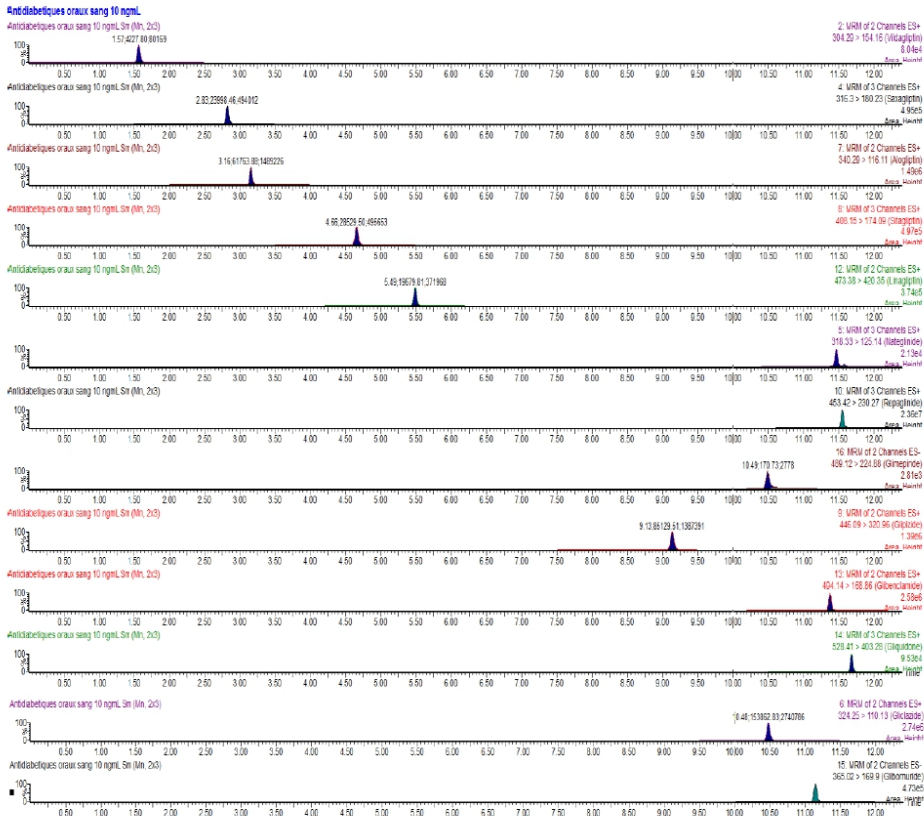
Figure 1. Chromatogrammes des transitions quantitatives pour un échantillon de sang contenant 10 ng/mL de chaque analyte.
