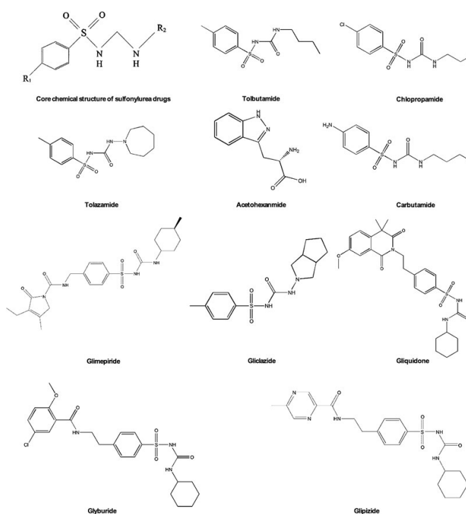
Figure 3. Structures chimiques des sulfamides hypoglycémiantes [38]
