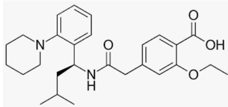
Figure 5. Structure chimique du répaglinide
