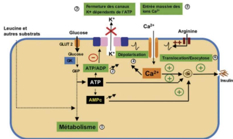
Figure 13. Mécanisme de sécrétion de l'insuline [43]
