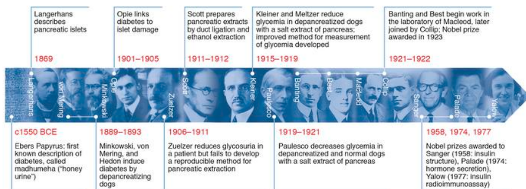
Figure 15. Histoire de la découverte de l'insuline au premier séquençage de l'insuline [28]
