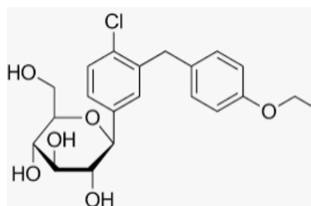
Figure 9. Structure chimique de la dapagliflozine
