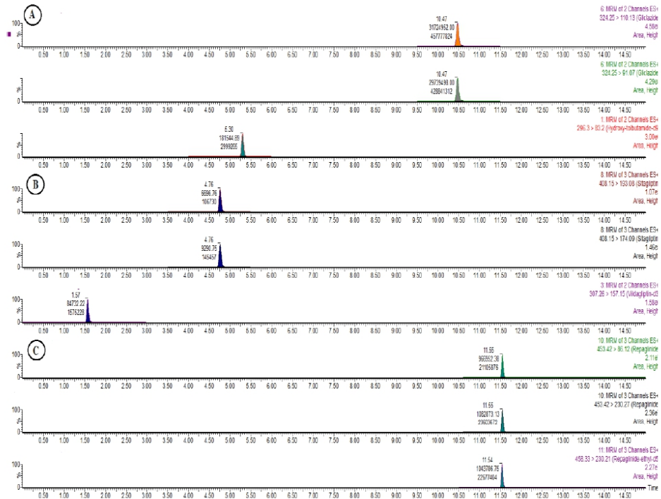
Figure 2. Chromatogrammes des transitions ioniques d'échantillons de sang postmortem contenant a) 2 transitions de gliclazide et 1 transition de l'IS (hydroxy tolbutamide-d9), la concentration était de 3000 ng/mL ; b) 2 transitions de sitagliptine et 1 transition de l'IS (vildagliptin-d3), la concentration était de 251 ng/mL ; c) 2 transitions de repaglinide et 1 transition de l'IS (repaglinide éthyl-d5), la concentration était de 15 ng/mL.
