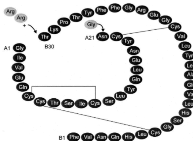
Figure 17. Structure de l'insuline glargine, insuline à durée prolongée [46]
