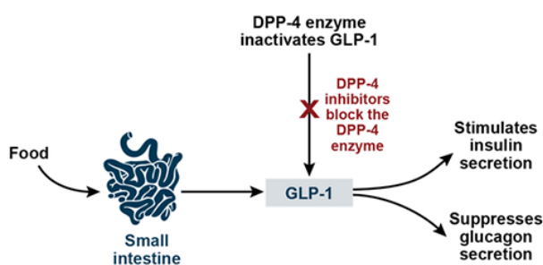
Figure 7. Mécanisme d'action des gliptines [41]
