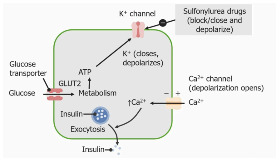
Figure 4. Mécanisme d'action des sulfamides hypoglycémiantes [39]
