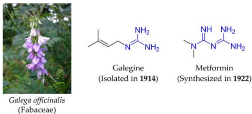
Figure 1. Structures chimiques de la metformine et de la galéguine [36]
