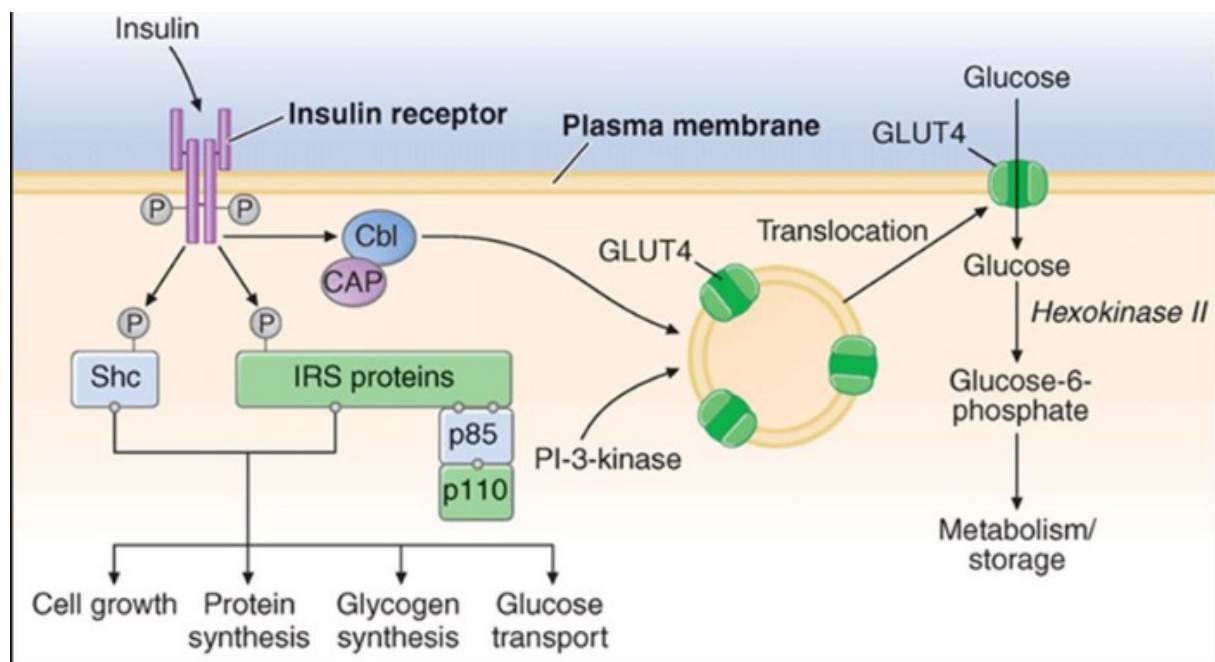
Figure 14. Mécanisme d'action de l'insuline [44]
