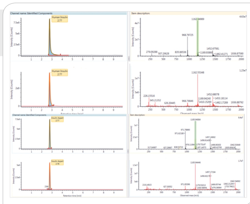
Figure 1 Chromatogrammes et spectres de l'insuline humaine et de l'insuline aspartate obtenus en LC-HRMS
