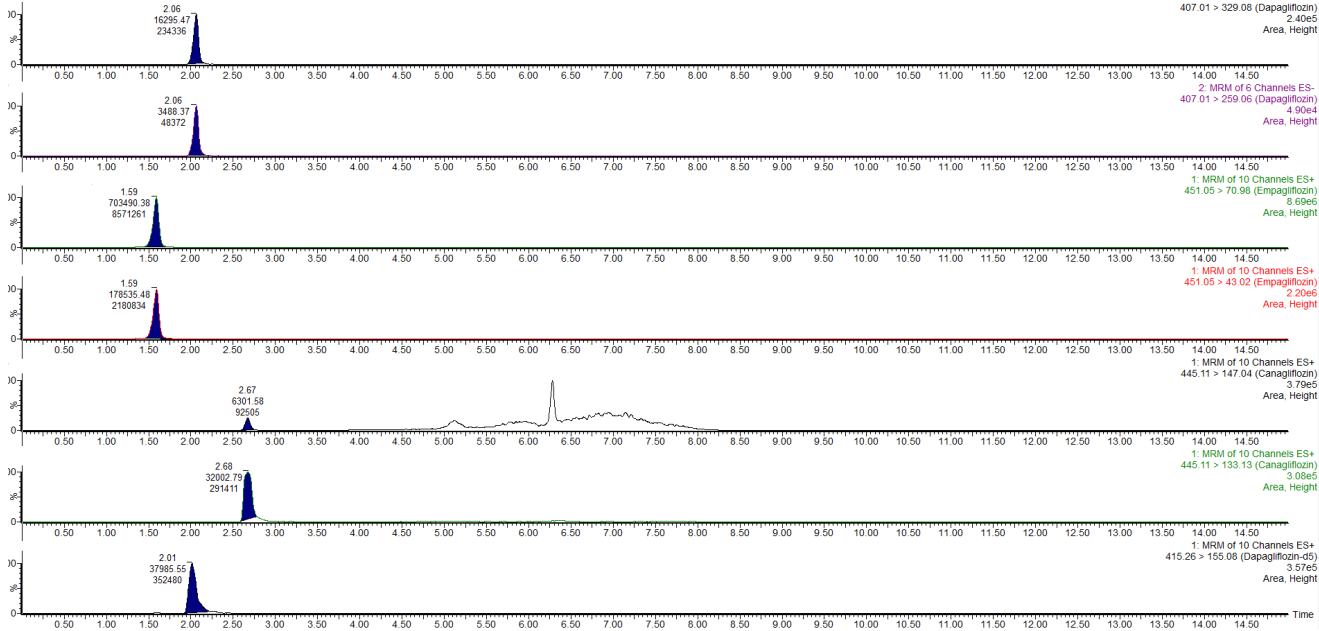
Figure 11. Chromatogrammes des transitions quantitatives et qualitatives pour un échantillon de sang contenant 100 pg/mg de chaque analyte
