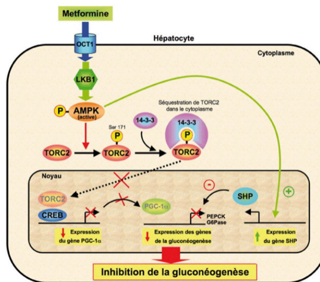
Figure 2. Mécanismes d'inhibition de la gluconéogenèse hépatique par la metformine [37]
