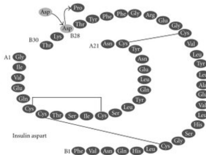
Figure 16. Structure de l'insuline aspart, insuline à action rapide [45]
