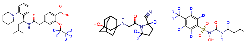
Figure 10. Répaglinide-éthyl-d5 (gauche), vildagliptine-d3 (milieu), hydroxy-tolbutamide-d9 (droite)
