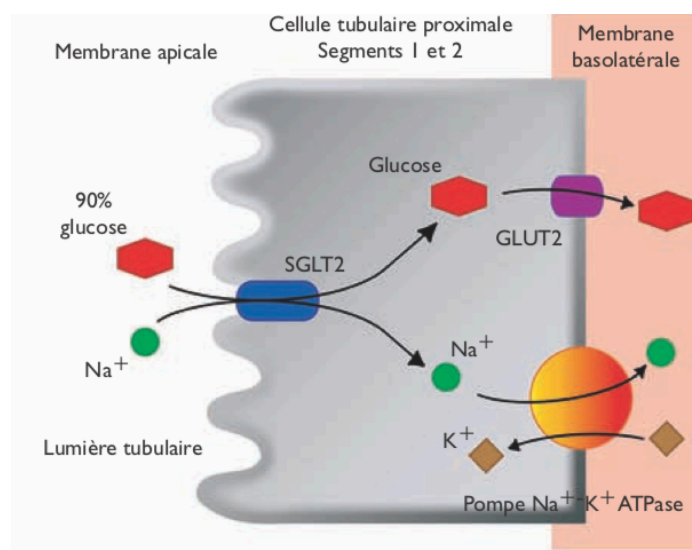
Figure 8. Mécanisme d'action des cotransporteurs SGLT-2 [42]
