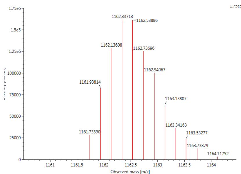
Figure 18. Spectre de l'ion pseudo-moléculaire m/z [M+5]^{5+} 1162.33713 de l'insuline humaine
