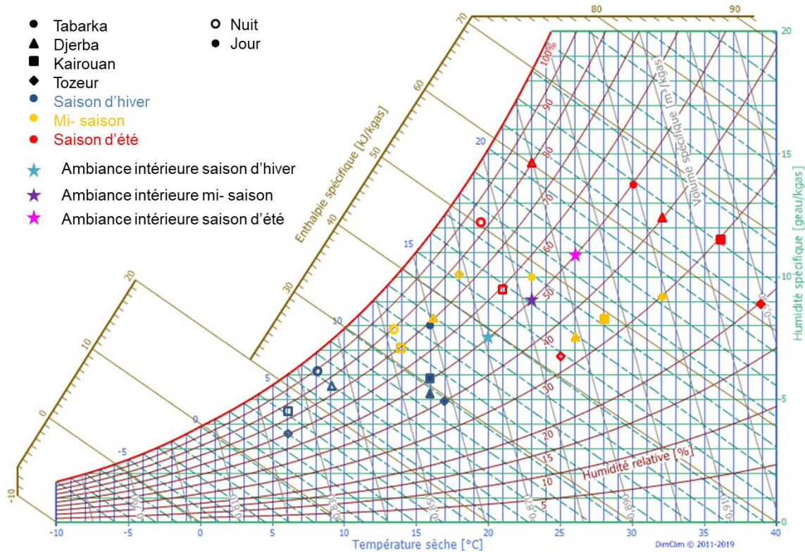
Figure II-38 : Températures et humidités relatives caractéristiques des villes tunisiennes pendant les différentes saisons
