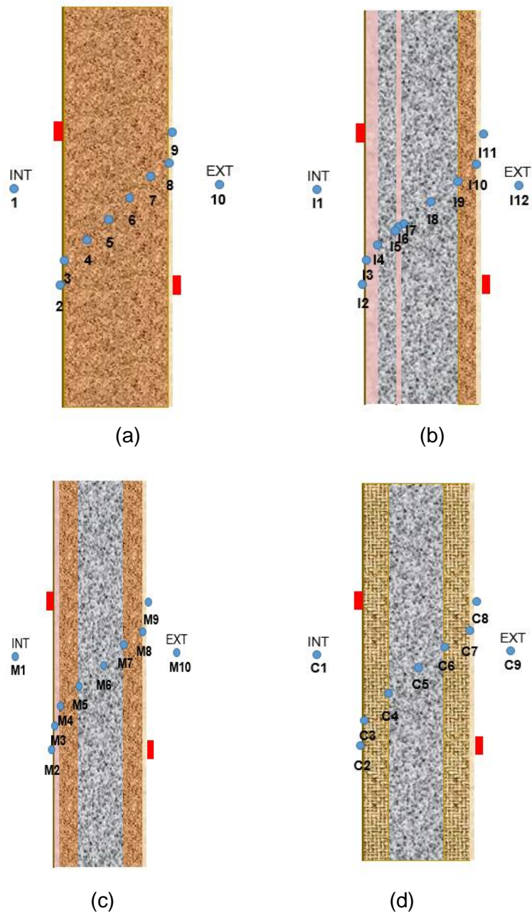
Figure II-27 : Implantation des capteurs dans les parois : (a) Paroi Terre-Chanvre, (b) Paroi ISOBIO, c) Paroi Maïs : en panneaux de PVA-chanvre avec un parement intérieur en résidus de rafles de maïs, (d) Paroi Colza : en panneaux de résidus de paille de colza
