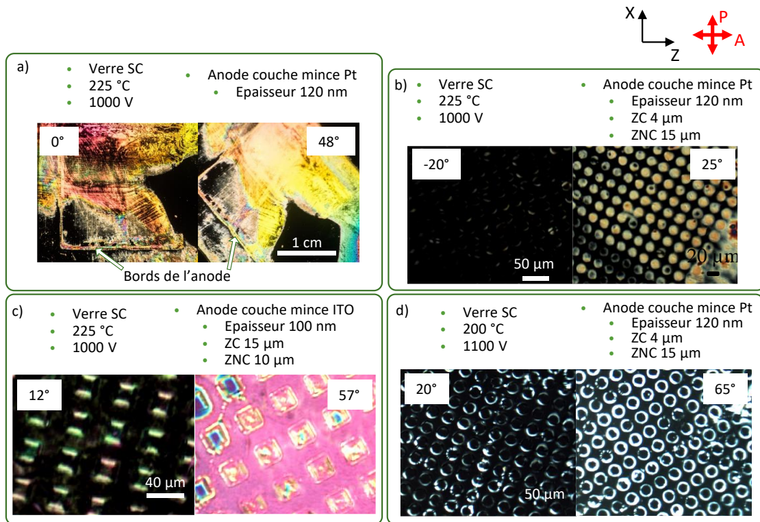
Figure 5-3. Observations macroscopiques a) et en microscopie optique b), c), d) en lumière transmise polarisée de plusieurs cellules à CL utilisant des verres sodo-calciques polés sous différentes conditions. Les conditions de traitement sont indiquées sur la figure, avec ZC = zone conductrice et ZNC = zone non-conductrice.
