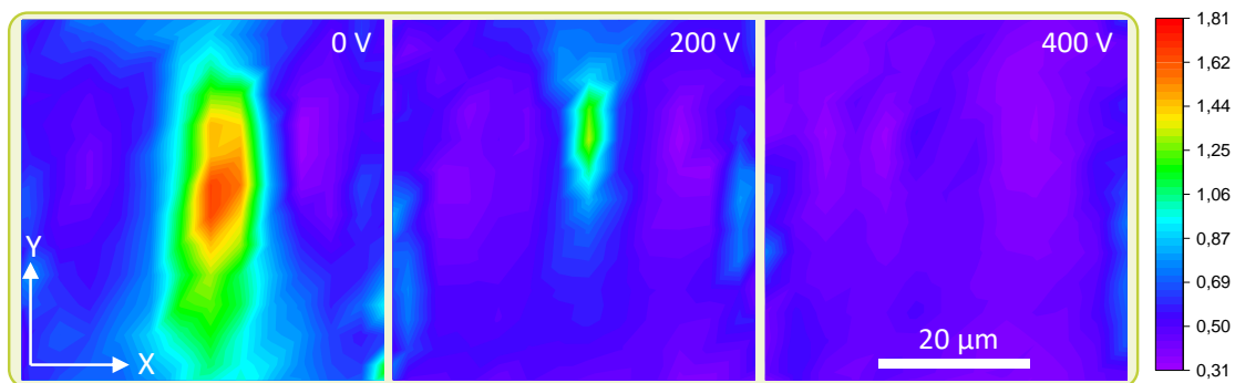
Figure 4-20. Rapport R = I_{zz}/I_{xx} pour un capillaire de 60 \mu\text{m} pour différentes valeurs de tension
