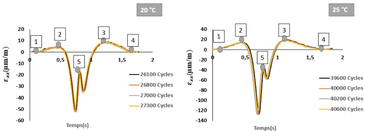
Figure II-47 : Analyse de la reproductibilité des signaux longitudinaux relevés au dessus de la couche résiduelle
