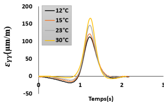
Figure III-7 : Signaux de déformations transversales en surface (à h=0 ; y=60\text{cm} ) pour l'Agreco
