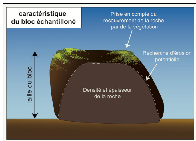
Figure 47: Caractéristiques à prendre en compte pour chaque bloc échantillonné sur le terrain dans le but d'obtenir un âge d'exposition.
