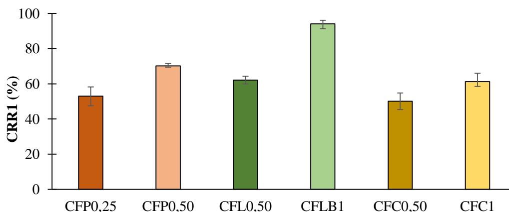
Figure IV-13: Le CRR1 des formulations cimentaires fibrées (essais sur moules avec surélévations)
