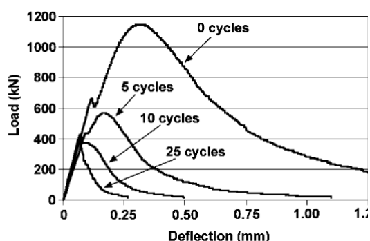
Figure I-40: Effet des cycles de vieillissement sur le comportement mécanique en flexion 3 points de ciment renforcé par des fibres de conifères (Mohr et al., 2005)
