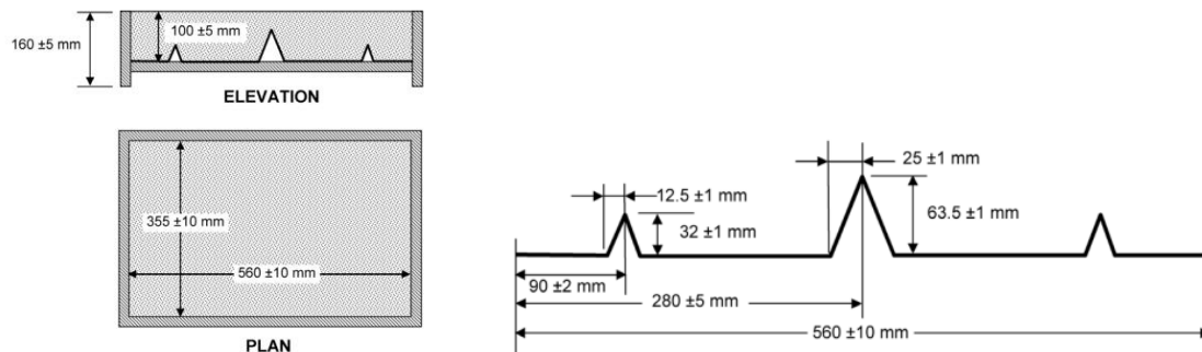
Figure IV-2: Les caractéristiques du moule prismatique et des surélévations métalliques selon la norme (ASTM C1579, 2006)
