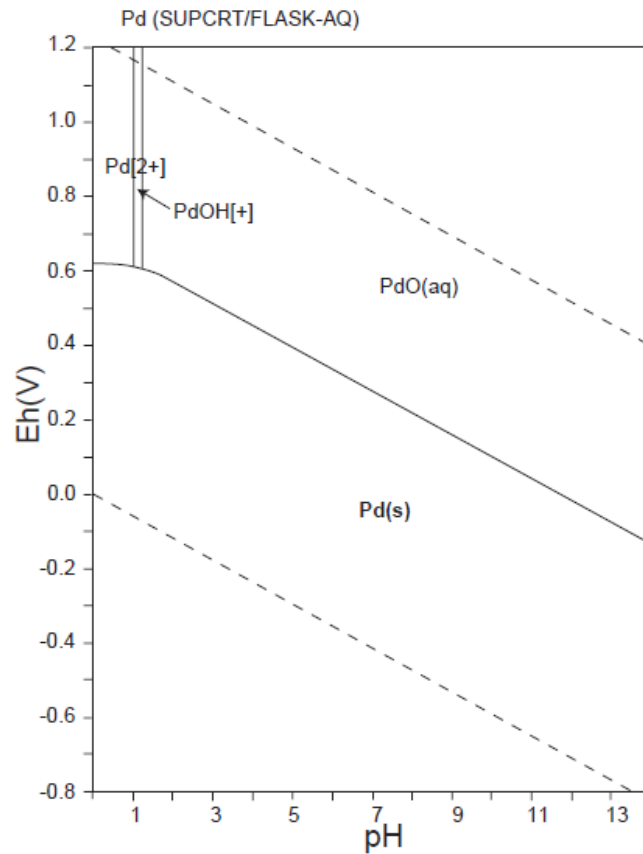
Figure 23 : diagramme Eh-pH du système Pd-O-H calculé à 298 K et 10 5 Pa pour \sum Pd = 10^{-10} \text{ mol.kg}^{-1} [118].
