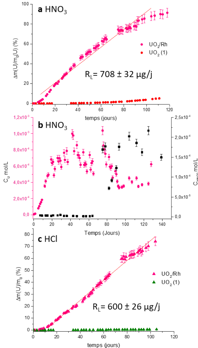
Figure 89 : évolution de la perte de masse relative en uranium lors de la dissolution de \text{UO}_2/\text{Rh} (●) et de \text{UO}_2 (●) dans \text{HNO}_3 0,1 M à 60°C (a). Evolution de la concentration en uranium (○) et en \text{HNO}_2 (■) lors de la dissolution de \text{UO}_2/\text{Rh} dans \text{HNO}_3 0,1 M à 60°C (b) Evolution de la perte de masse relative pendant la dissolution de \text{UO}_2/\text{Rh} (▲) et de \text{UO}_2 (▲) dans \text{HCl} 0,1 M à 60°C (c).
