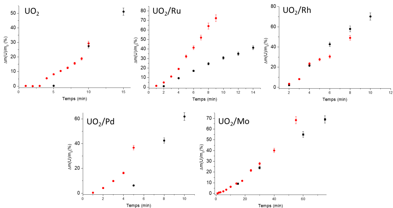
Figure 72 : évolutions des pertes de masse relatives relevées pour les différents systèmes modèles avec (●) et sans (●) suivi operando de dissolution ( \text{HNO}_3 4 M à 80°C).
