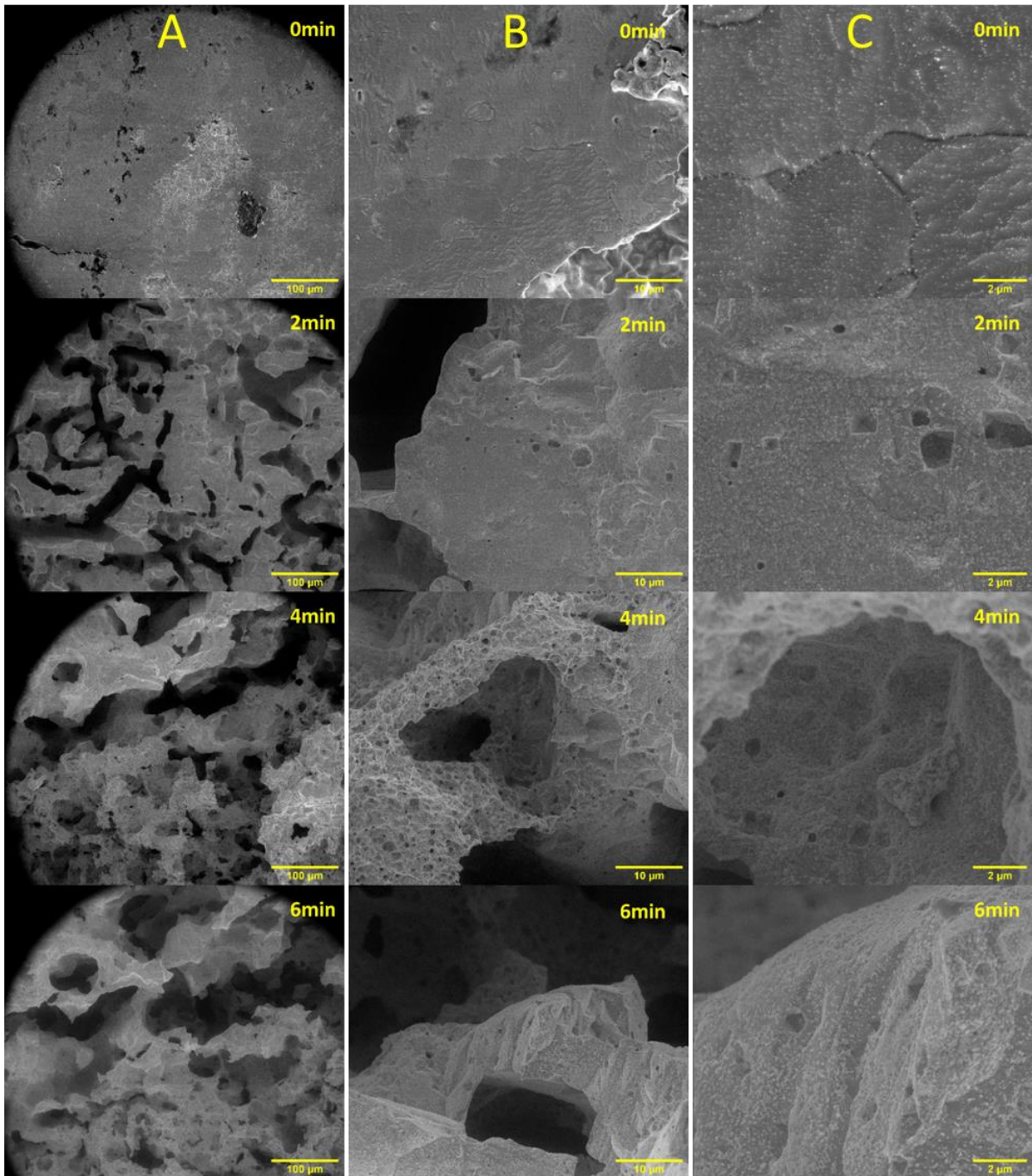
Figure 77 : suivi operando par MEBE de la dissolution d'un échantillon de \text{UO}_2/\text{Ru} dans \text{HNO}_3 4 M à 80^\circ\text{C} réalisé pour un grandissement de \times 250 (A), \times 2500 (B) et \times 10000 (C).
