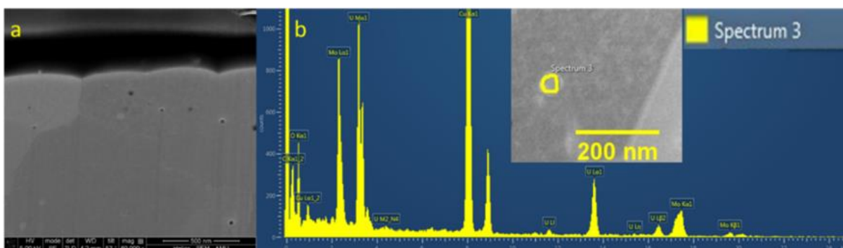
Figure 46 : image MEB de la lame FIB de \text{UO}_2/\text{Mo} (a) et spectre EDS d'une particule de Mo présente à l'intérieur de la pastille frittée (b).
