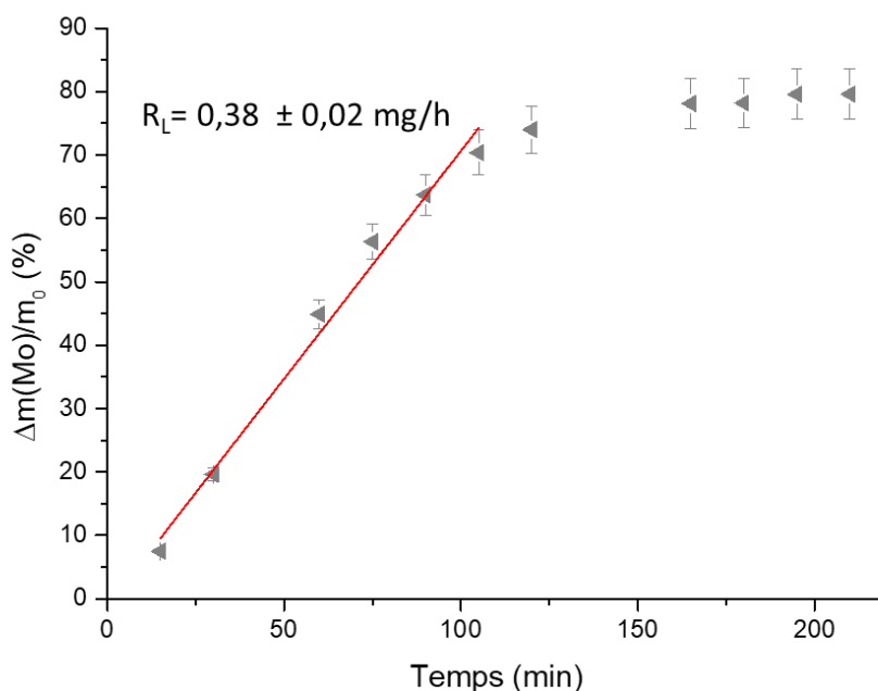
Figure 61 : évolution de la perte de masse relative en molybdène lors de la dissolution de \text{UO}_2/\text{Mo} dans \text{HNO}_3 4 M à 80^\circ\text{C} .
