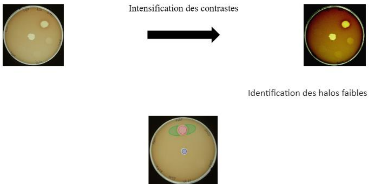
Figure_ 3: Identification des halos d'inhibition
