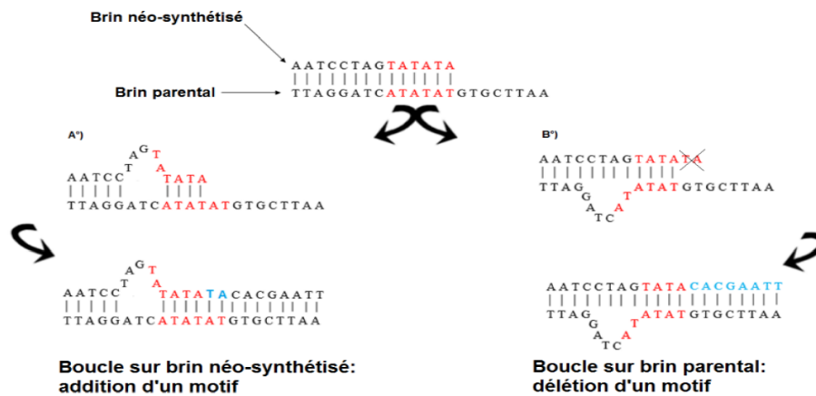
Figure 4: Modèle du Slipped Strand Mismatching (SSM)
