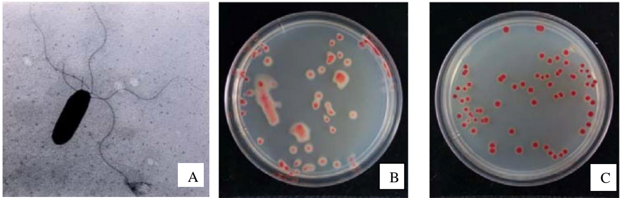
Figure 8: A) Image au microscope électronique du ceRs ; B) Colonies virulentes du ceRs sur un milieu contenant du TTC ; C) Colonies avirulentes du ceRs sur un milieu contenant du TTC.
