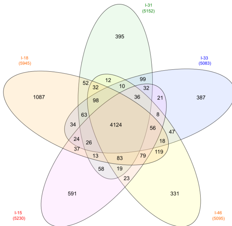
Figure_ 8: Diagramme de Venn représentant la distribution des 8014 familles de gènes du pangénome entre les différentes lignées génétiques
